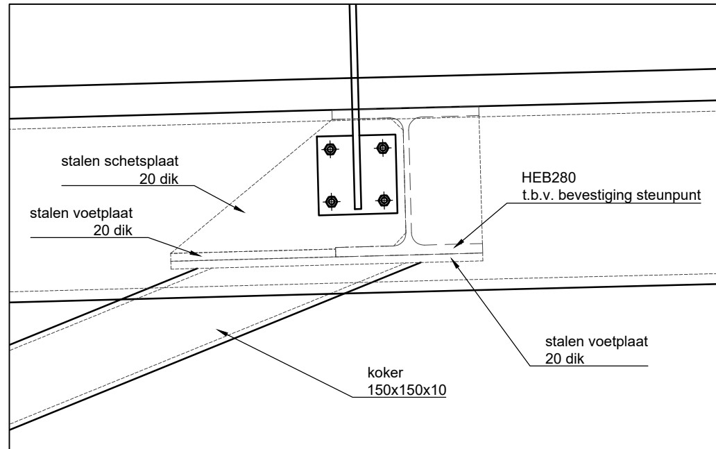
Detail 1 Schaal: 1:10
