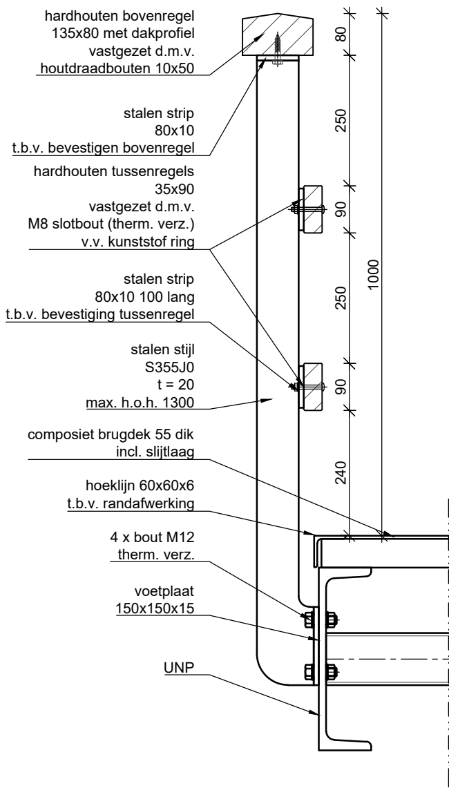
Detail leuning Schaal: 1:10
