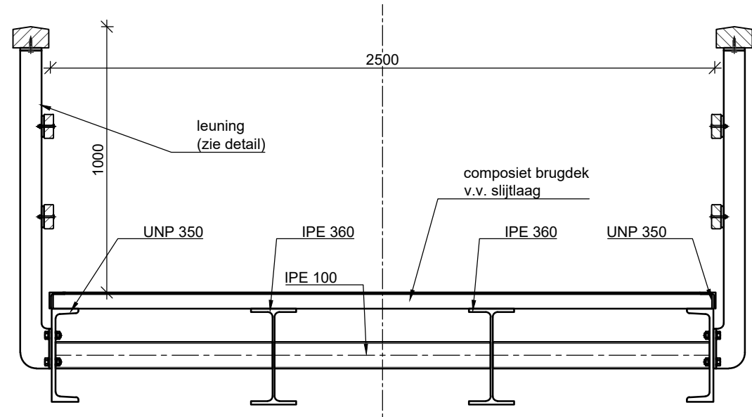
Doorsnede A-A Schaal: 1:20
