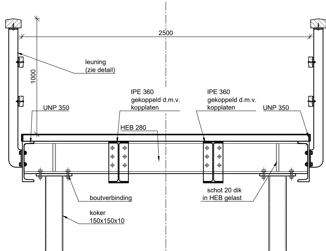
Doorsnede B-B Schaal: 1:20
