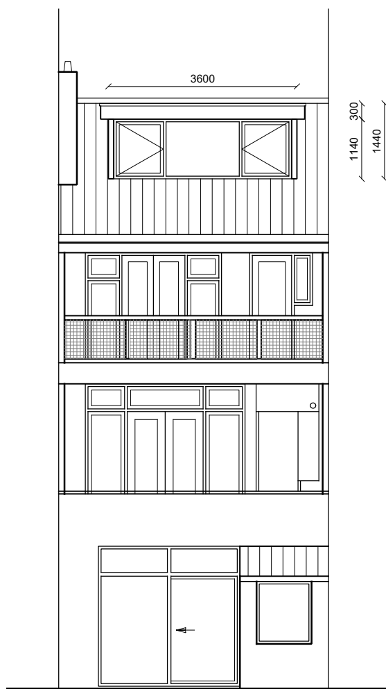
Achtergevel nieuw
