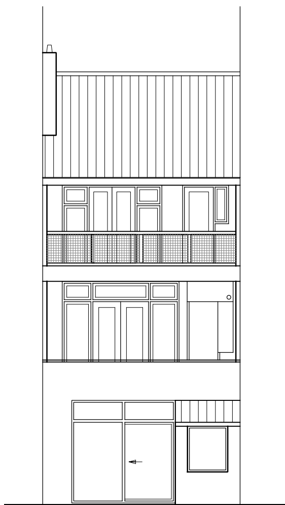
Achtergevel bestaand
