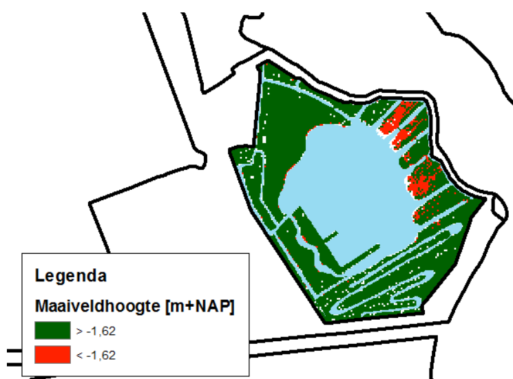
Figuur 4.2: Maaiveldhoogte (AHN3) rondom de Veerplas
