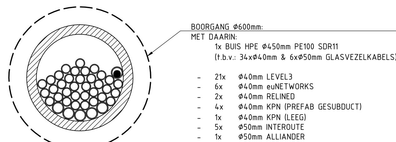
DOORSNEDEN BORING SCHAAL 1:10
