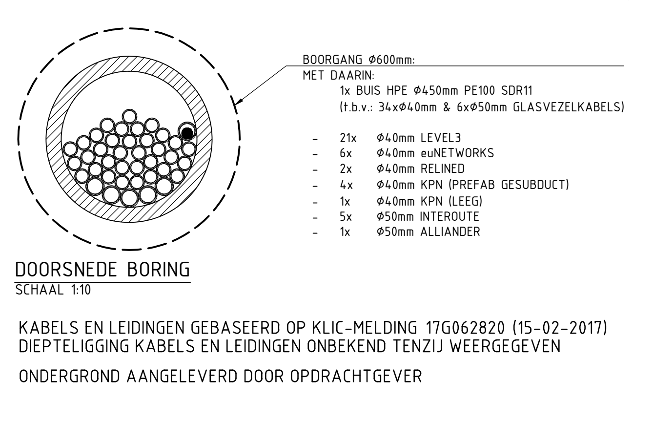
DOORSNEDEN BORING SCHAAL 1:10
