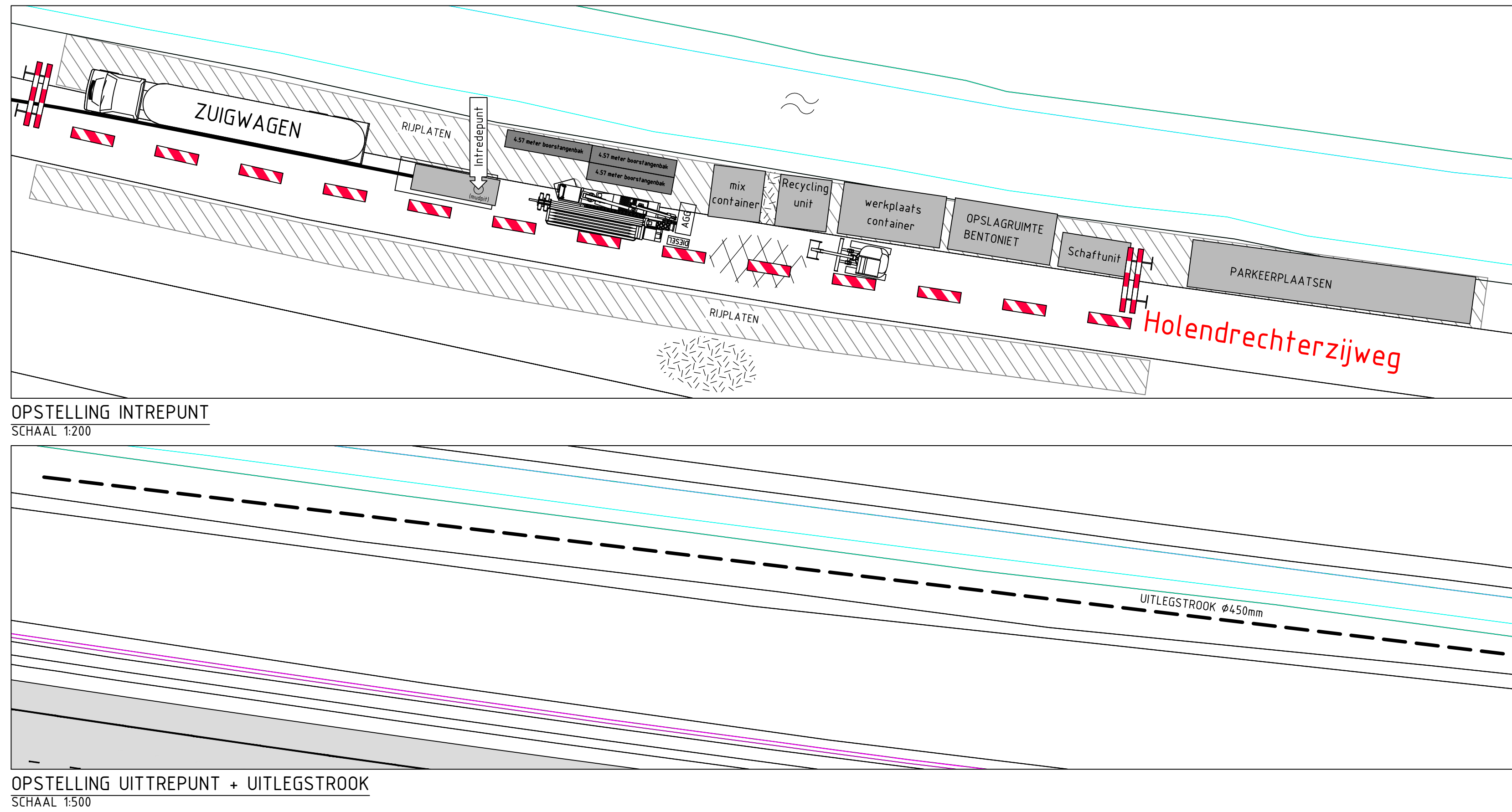
OPSTELLING INTREPUIT SCHAAL 1:200 OPSTELLING UITREPUIT + UITLEGSTROOK SCHAAL 1:500
