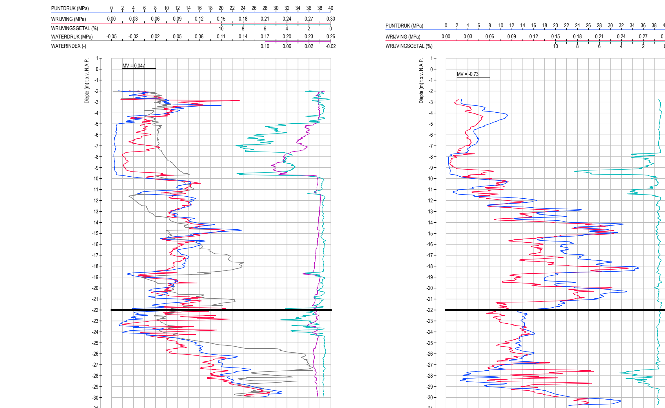
SONDERING S02 SCHAAL 1:200 SONDERING S01 SCHAAL 1:200
