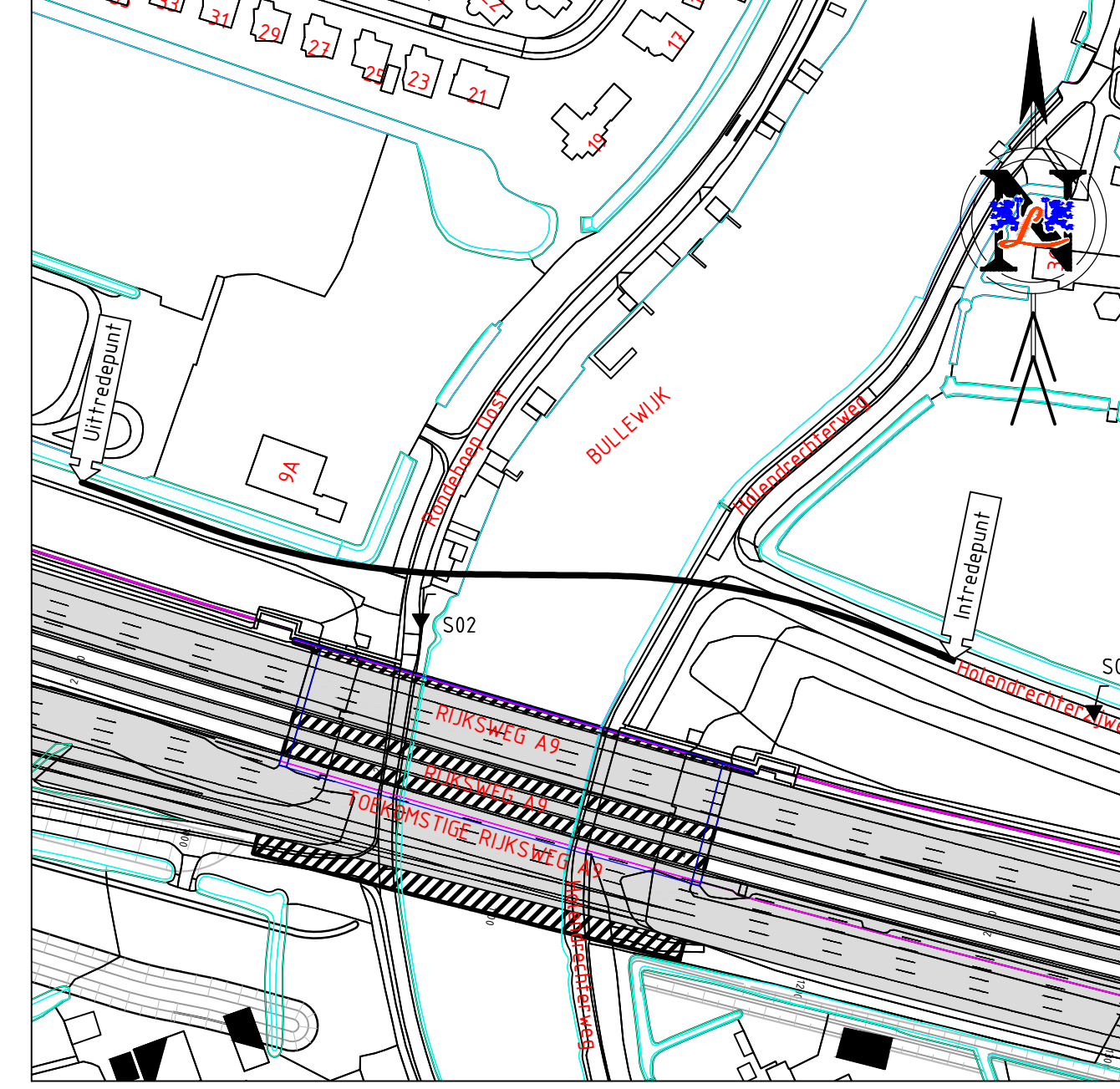
SITUATIE SCHAAL 1:2000
