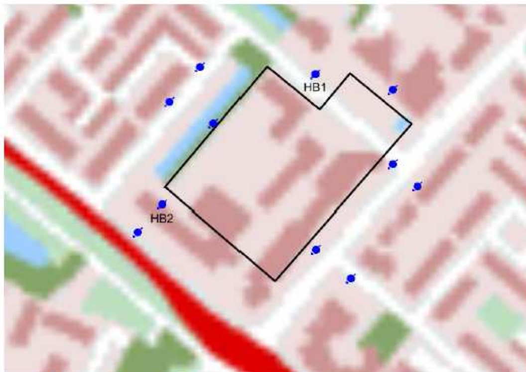
Afbeelding 5-1: Voorstel locaties monitoringspeilbuizen
