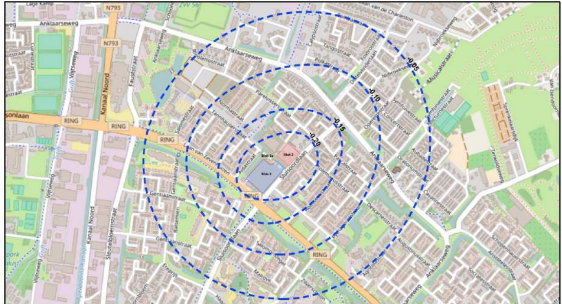
Figuur 4 – Verlaging grondwaterstand
