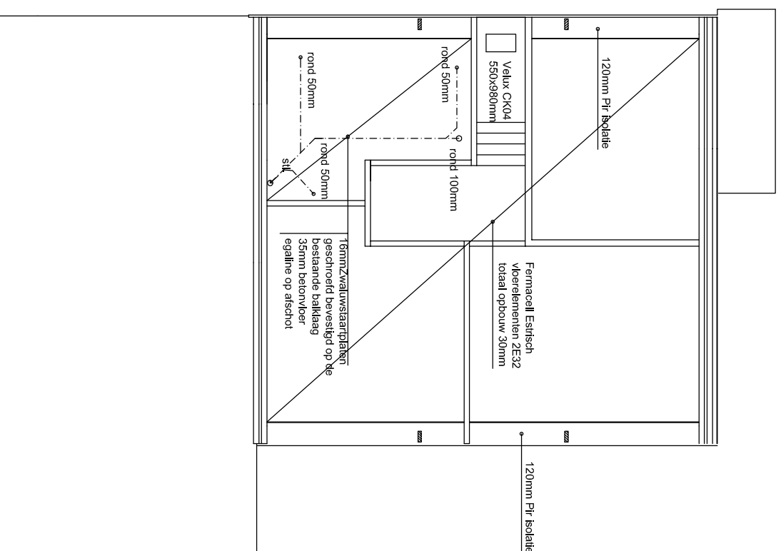
Gewijzigd vloerenplan verdieping
