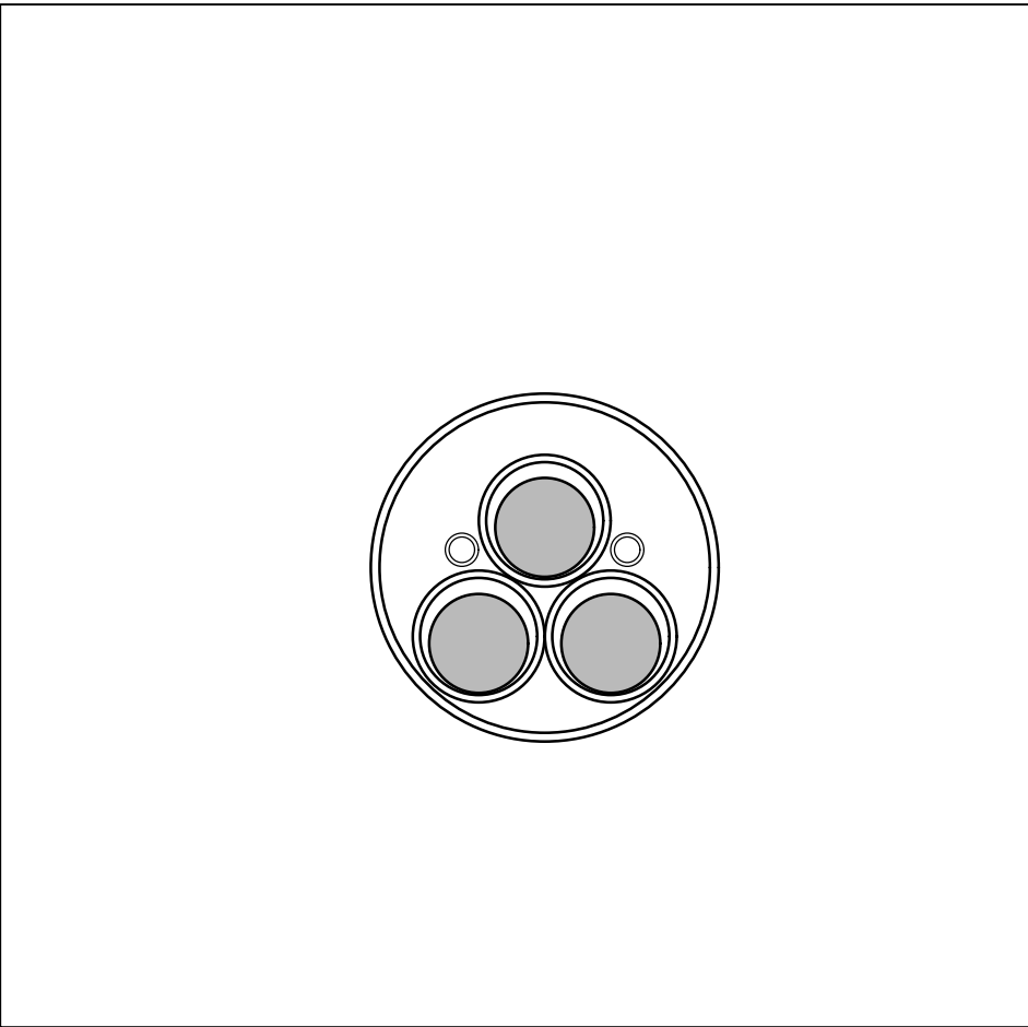
Doorsnede buizenpakket: 1x Wavin buis Ø420,8/400 met daarin 3x Flex buizen Ø160+ 2x gv-buisjes Ø40 schaal: 1:10
