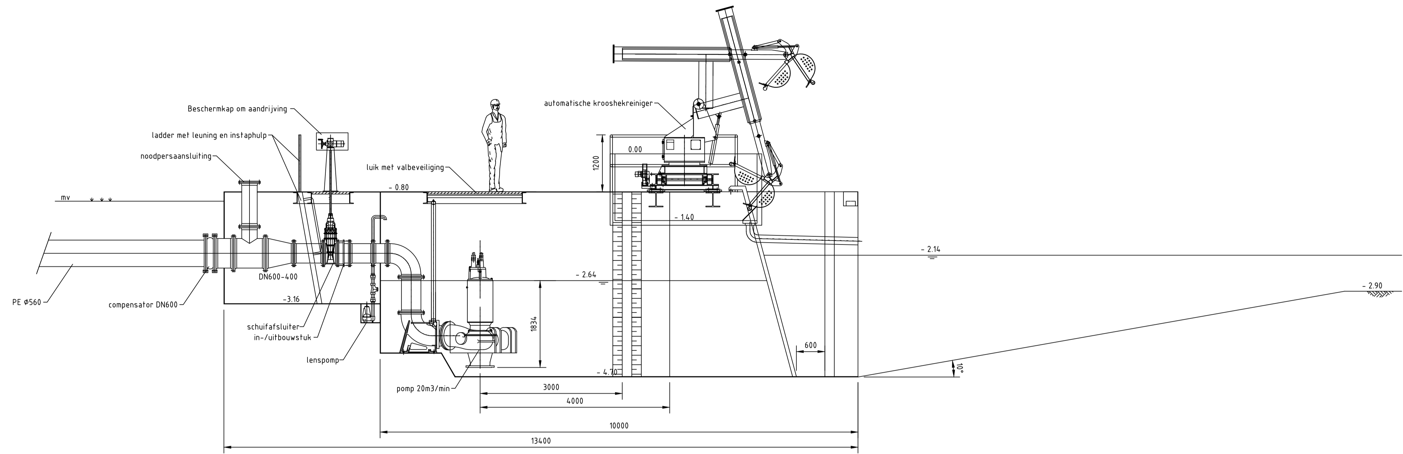
Doorsnede A-A
