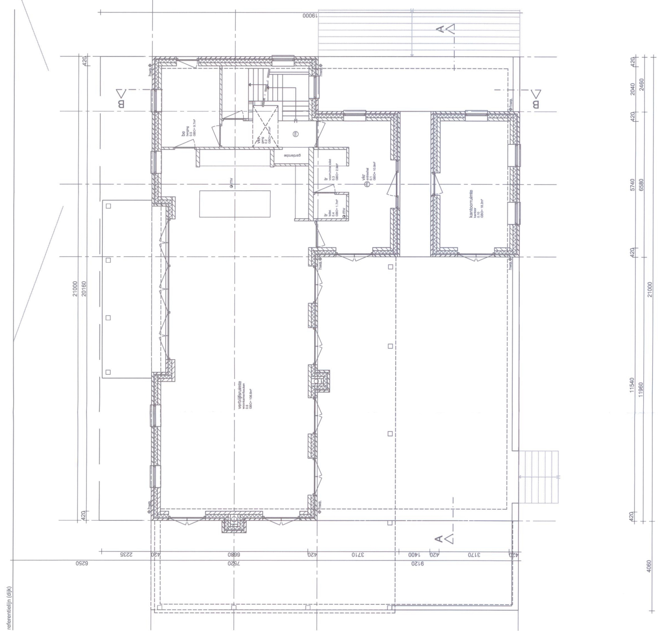
Begane grond
