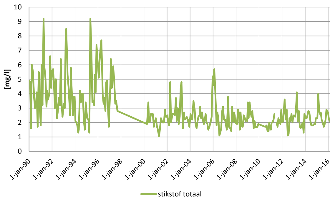
Figuur 3.20 Totaal-stikstof (mg/l) in de Reeuwijkse Plassen
