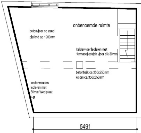
principeschets kelder
