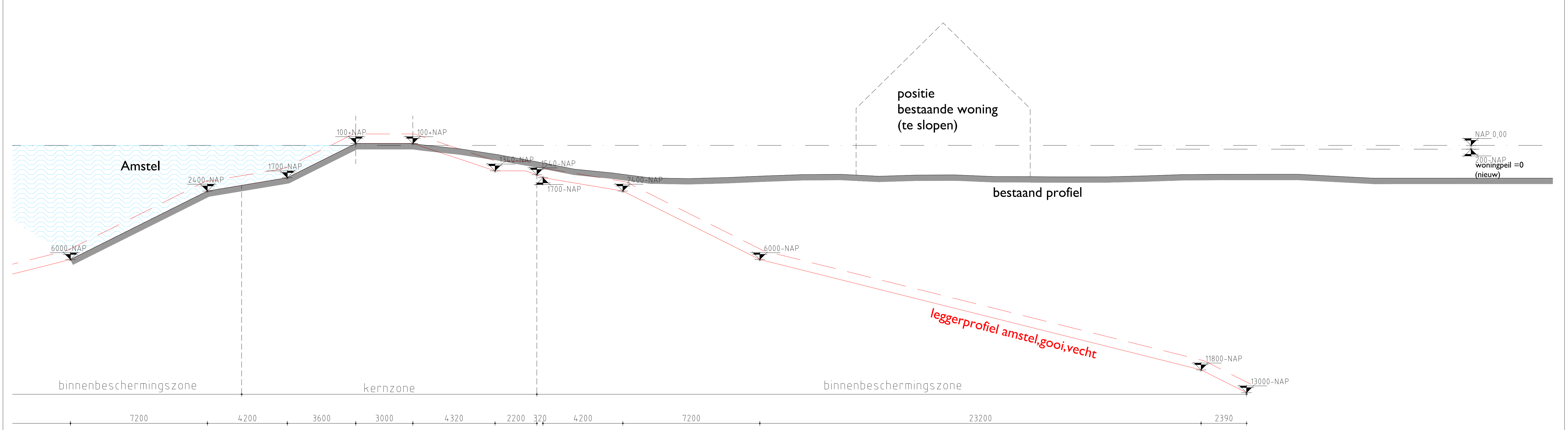
Terreindoorsnede A (bestaand)
