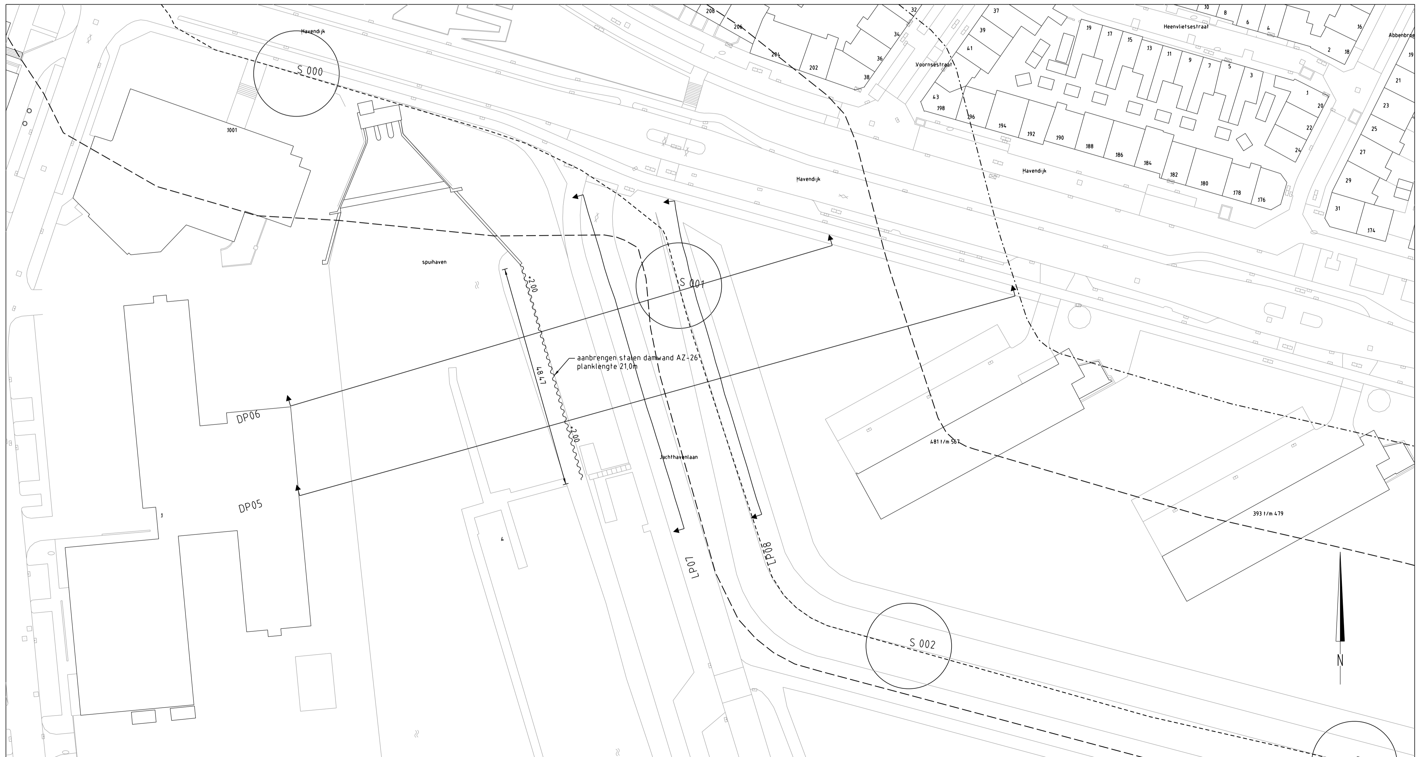
BOVENAANZICHT Schaal 1:500
