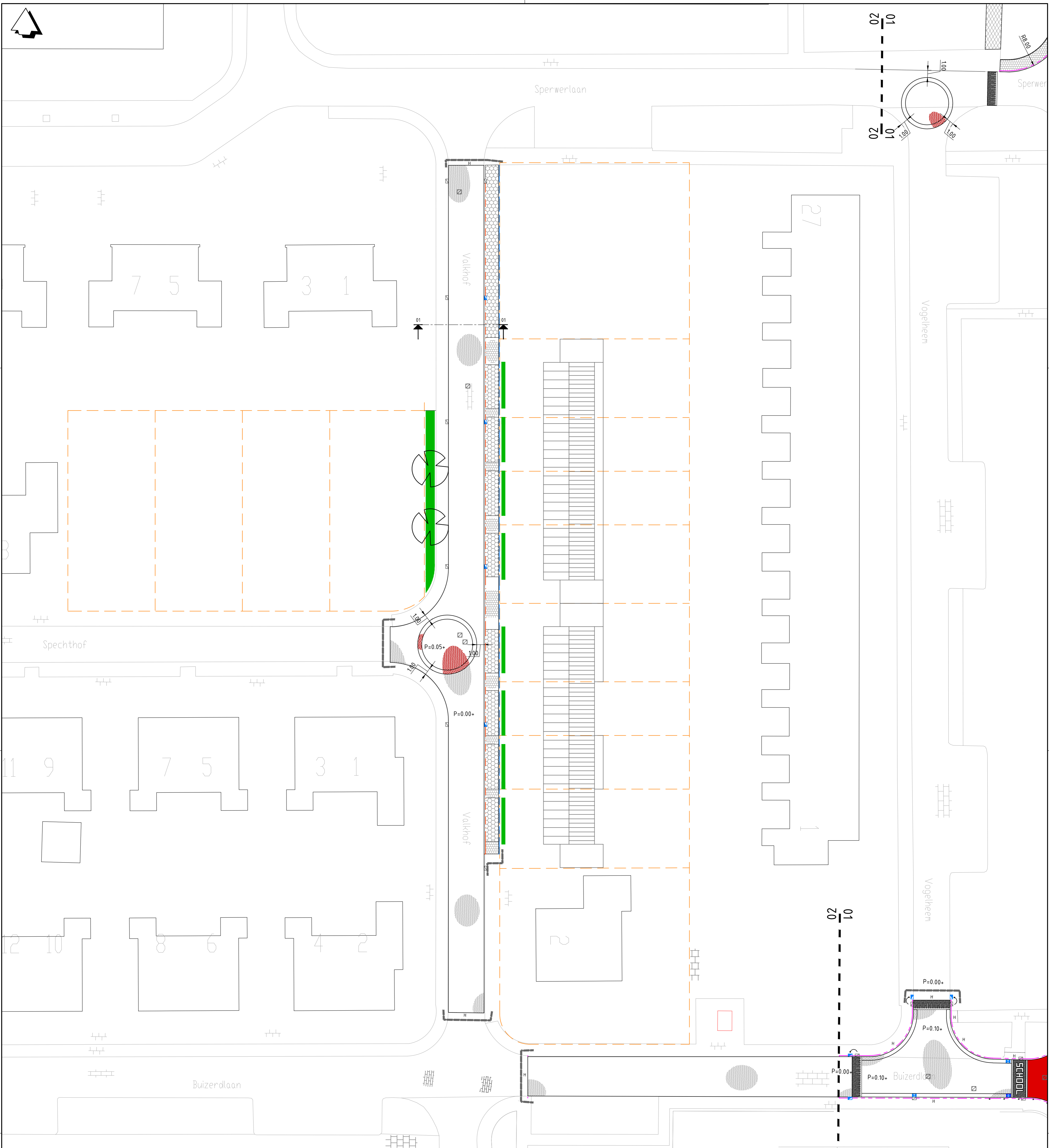
Situatie SWBS Pork SCHAAL 1 : 250
