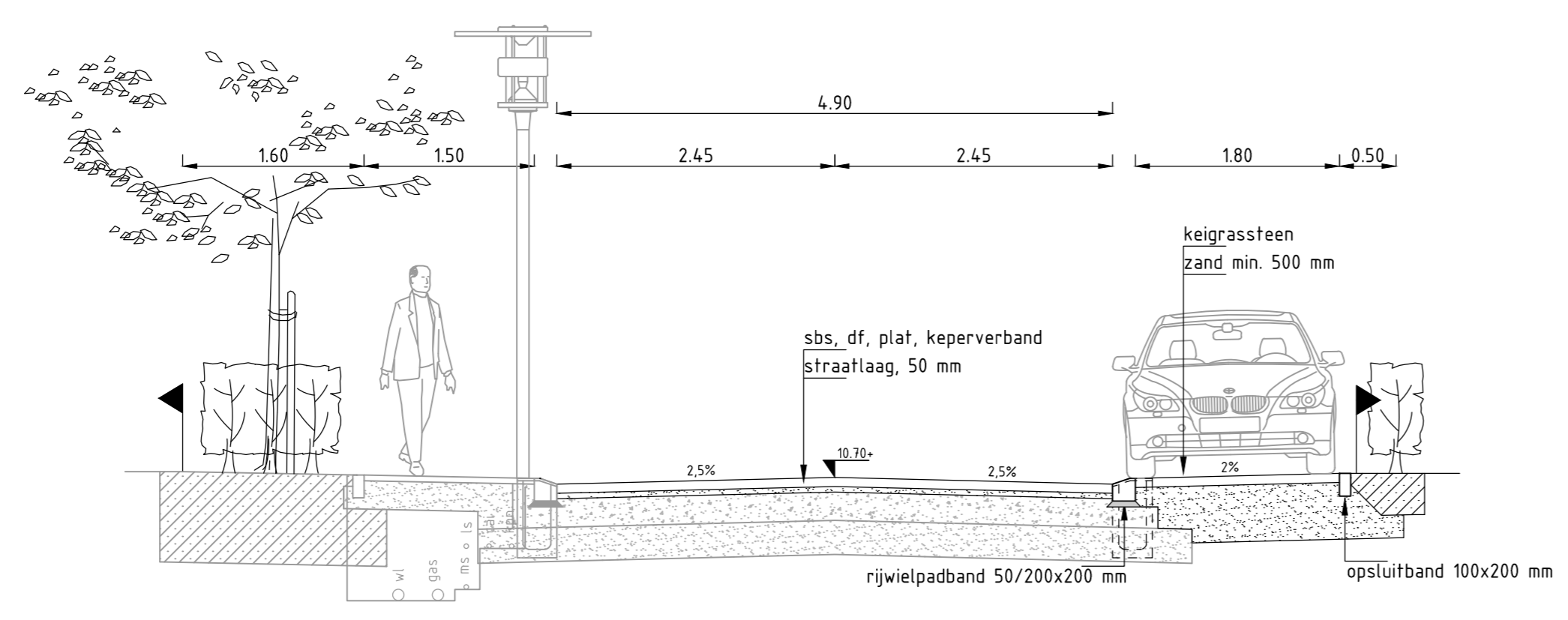
Profiel 1-1 SCHAAL 1 : 50
