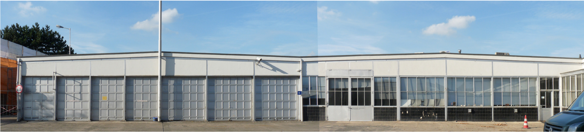
1. zuidoostgevel
