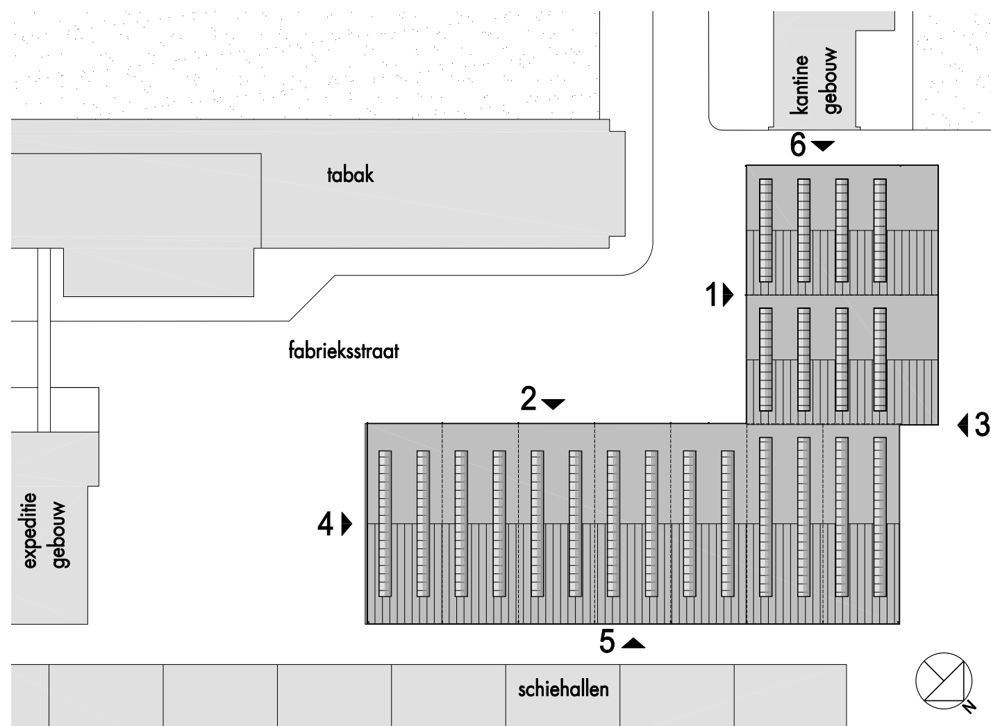
situatietekening
