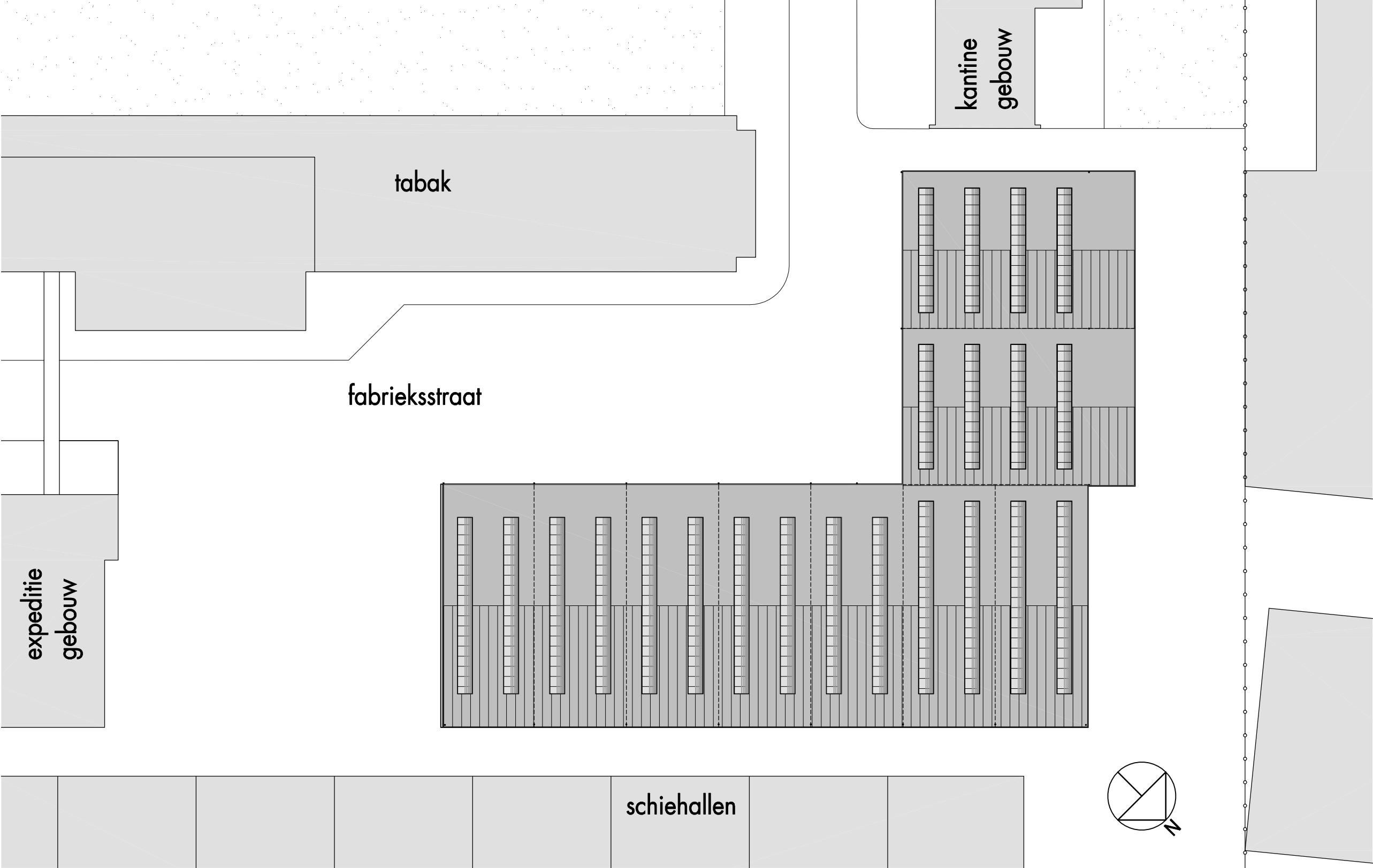
situatietekening
