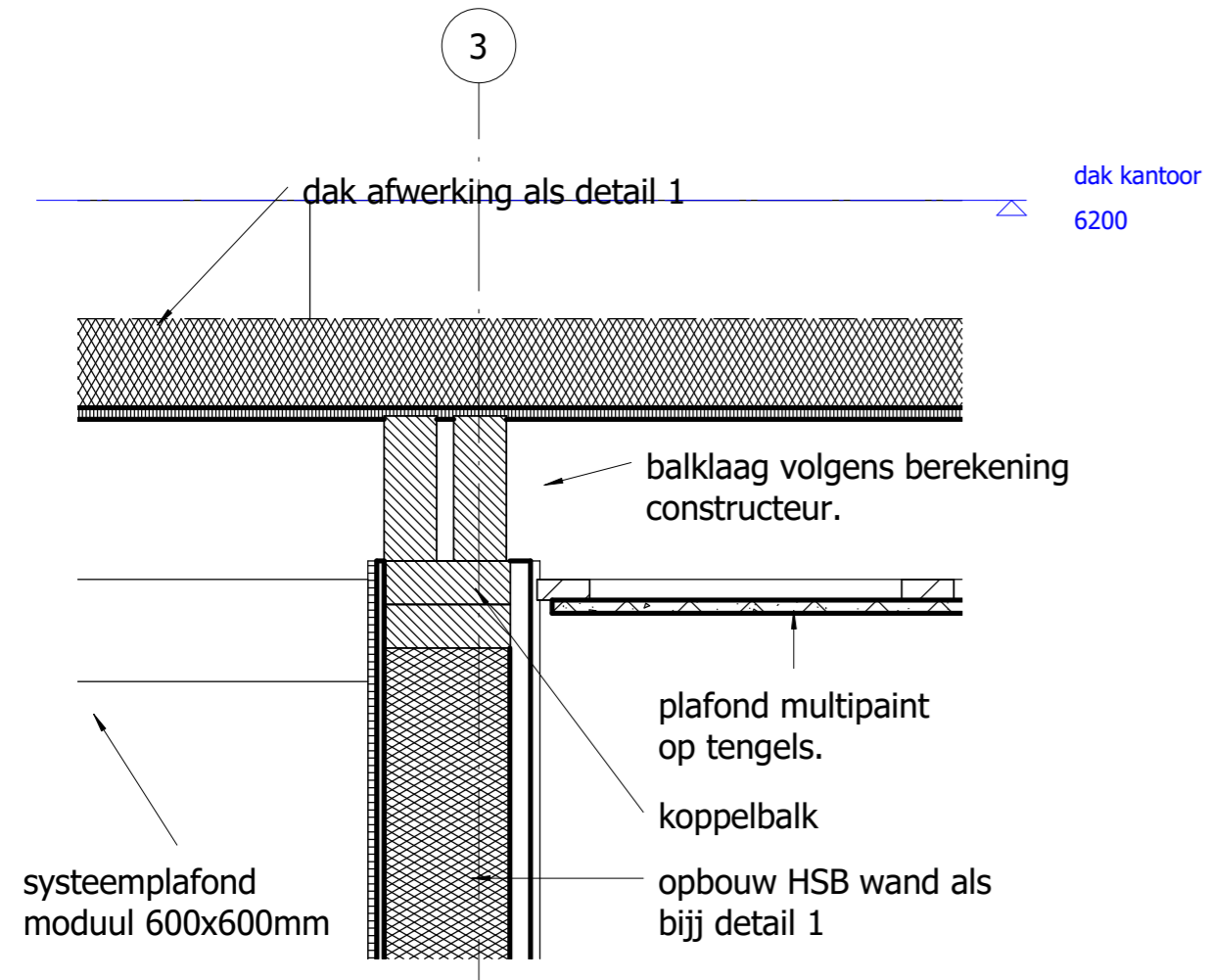
d3 detail 3 1 : 10
