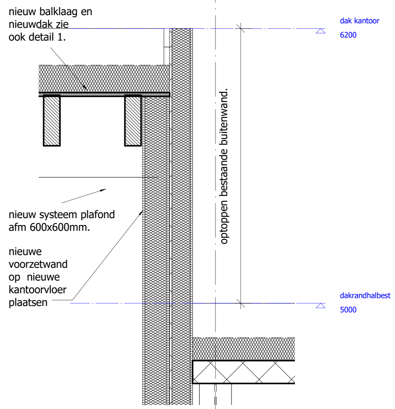
d6 detail 6 1 : 10
