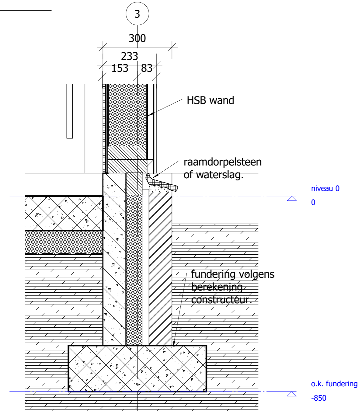
d3 detail 3 1 : 10
