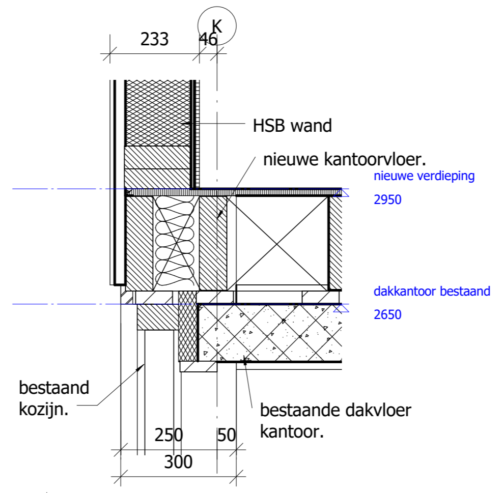
d7 detail 7 1 : 10
