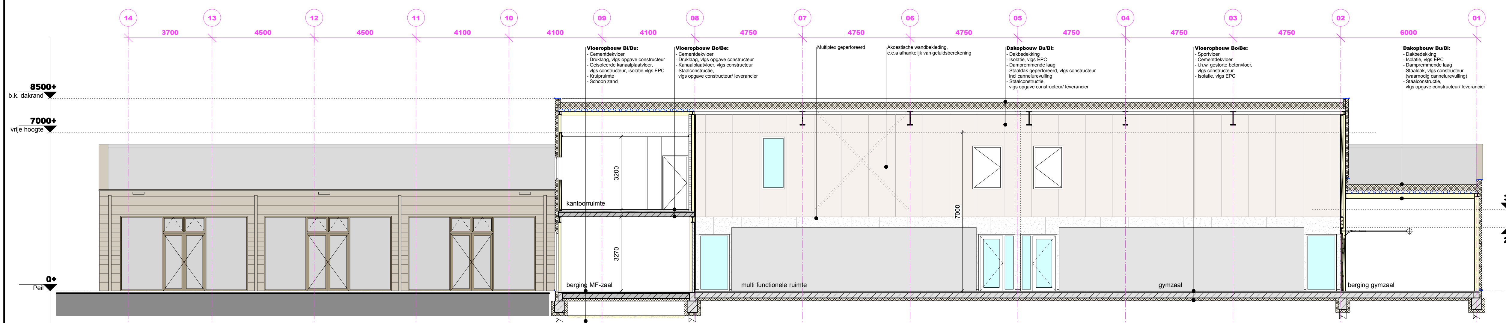
DOORSNEDE G-G
