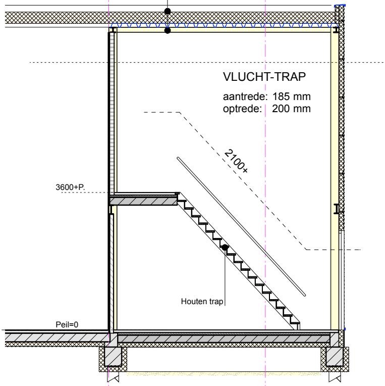
DOORSNEDE H
