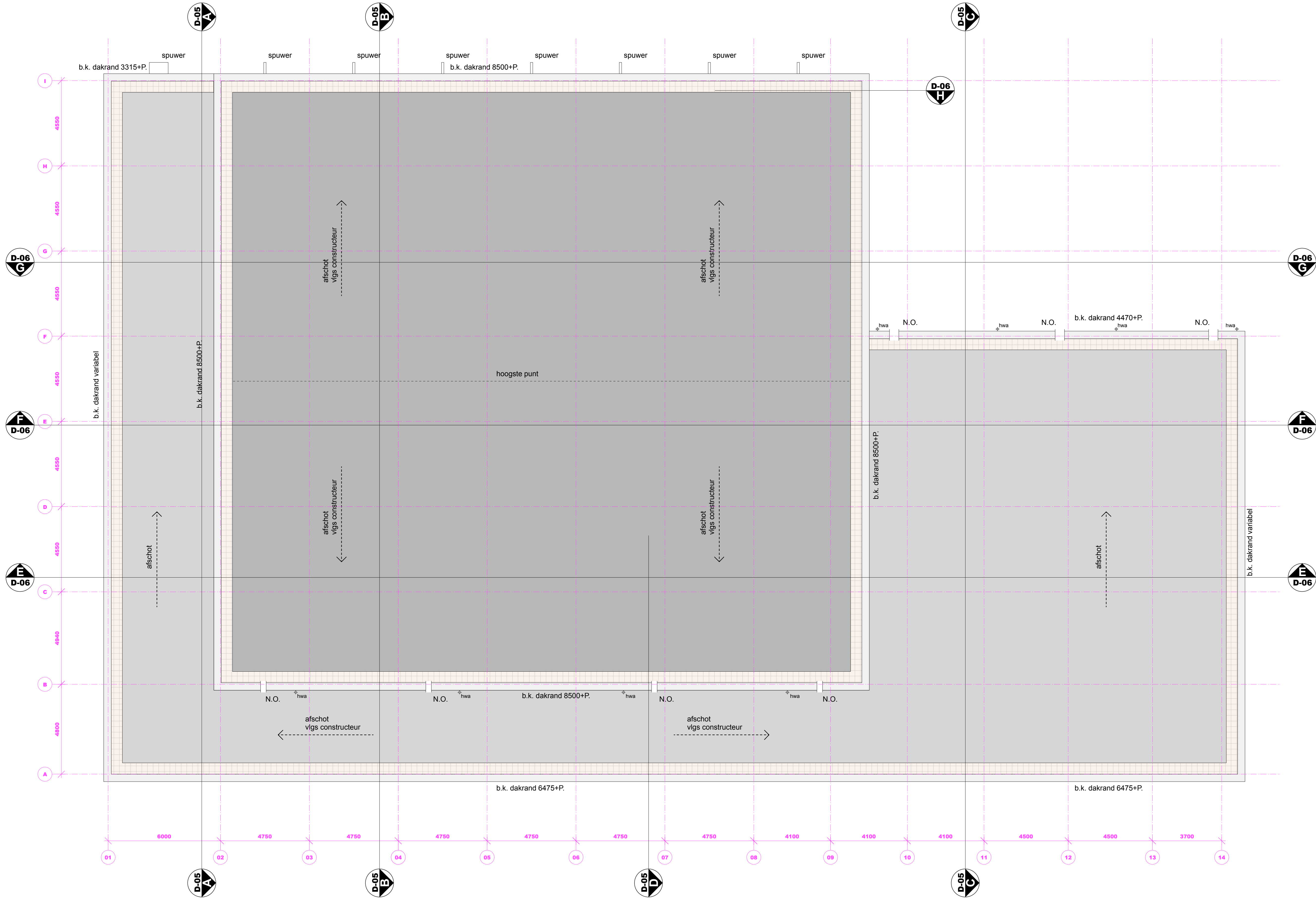
DAKOVERZICHT
