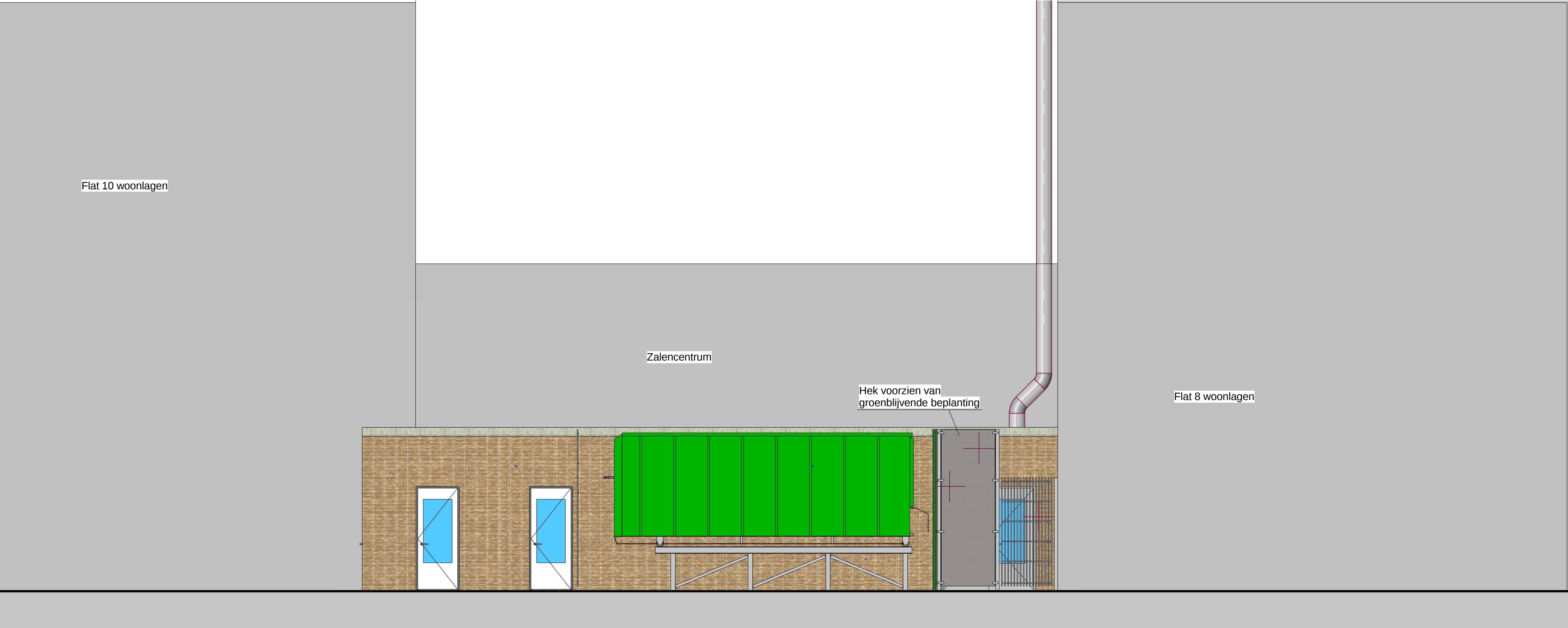
Gevelaanzicht toegang techniekrumte
