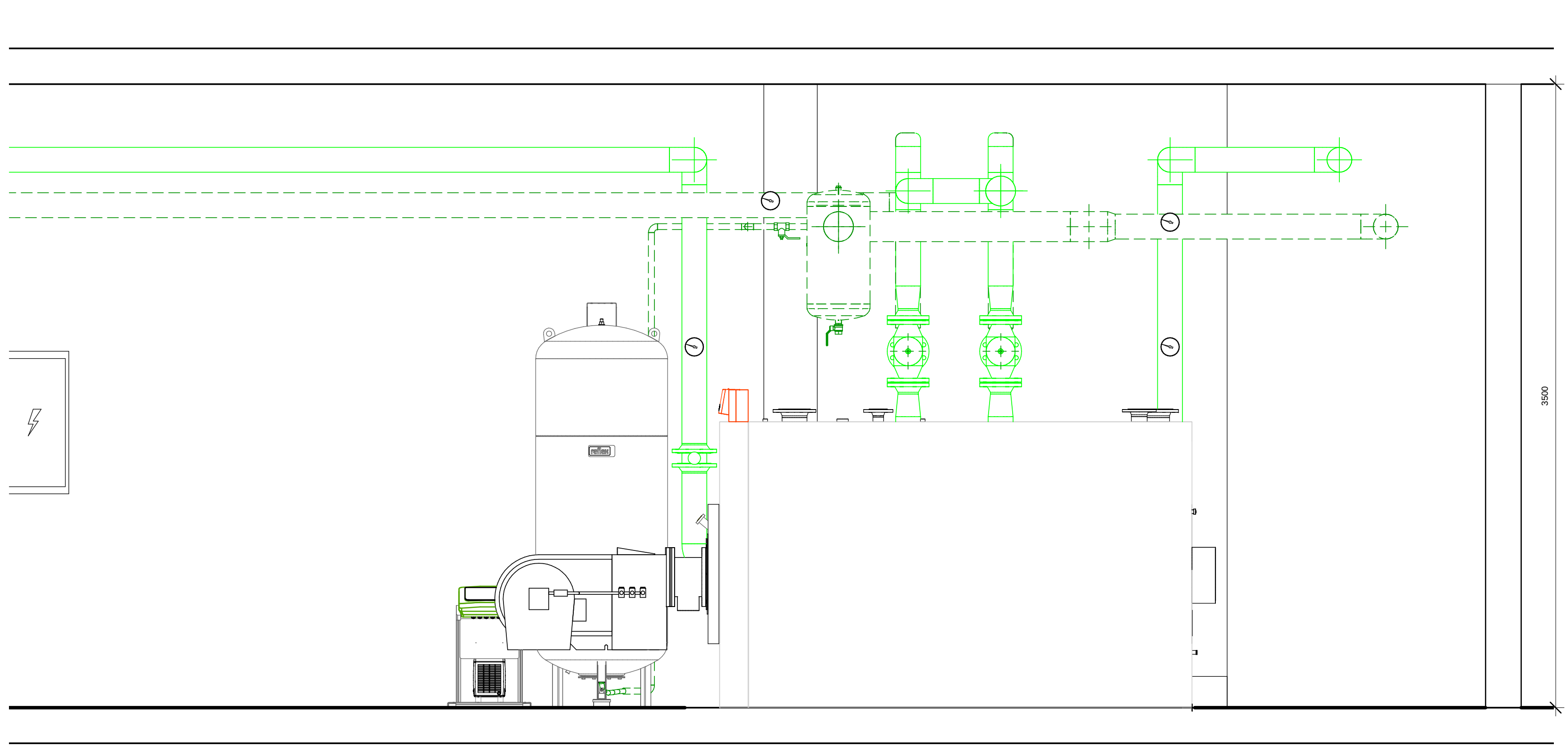
Doorsnede B-B 1 : 20
