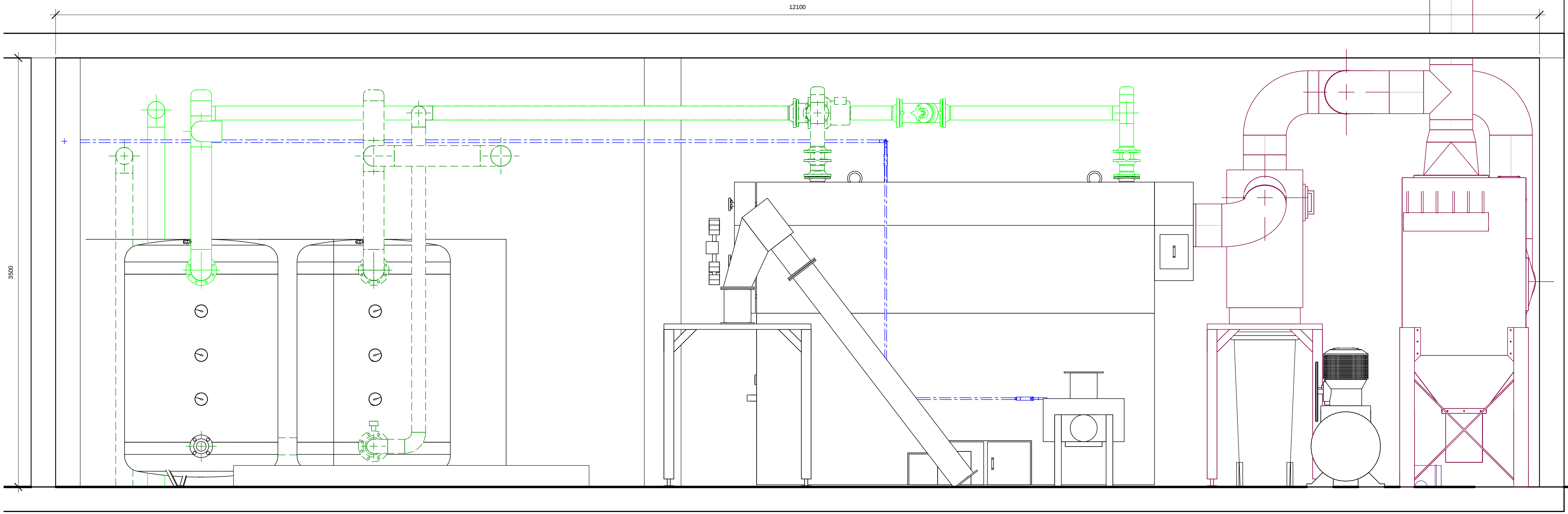
Doorsnede A-A 1 : 20
