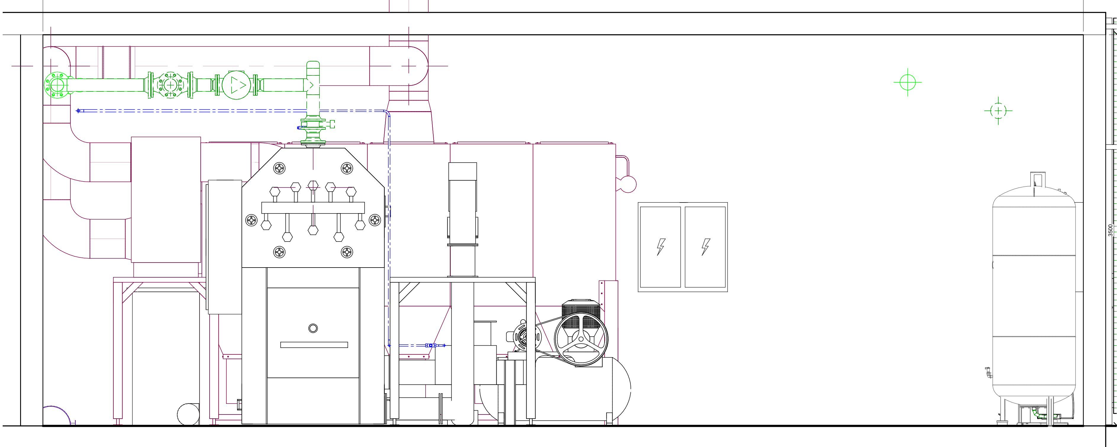
Doorsnede D-D 1 : 20
