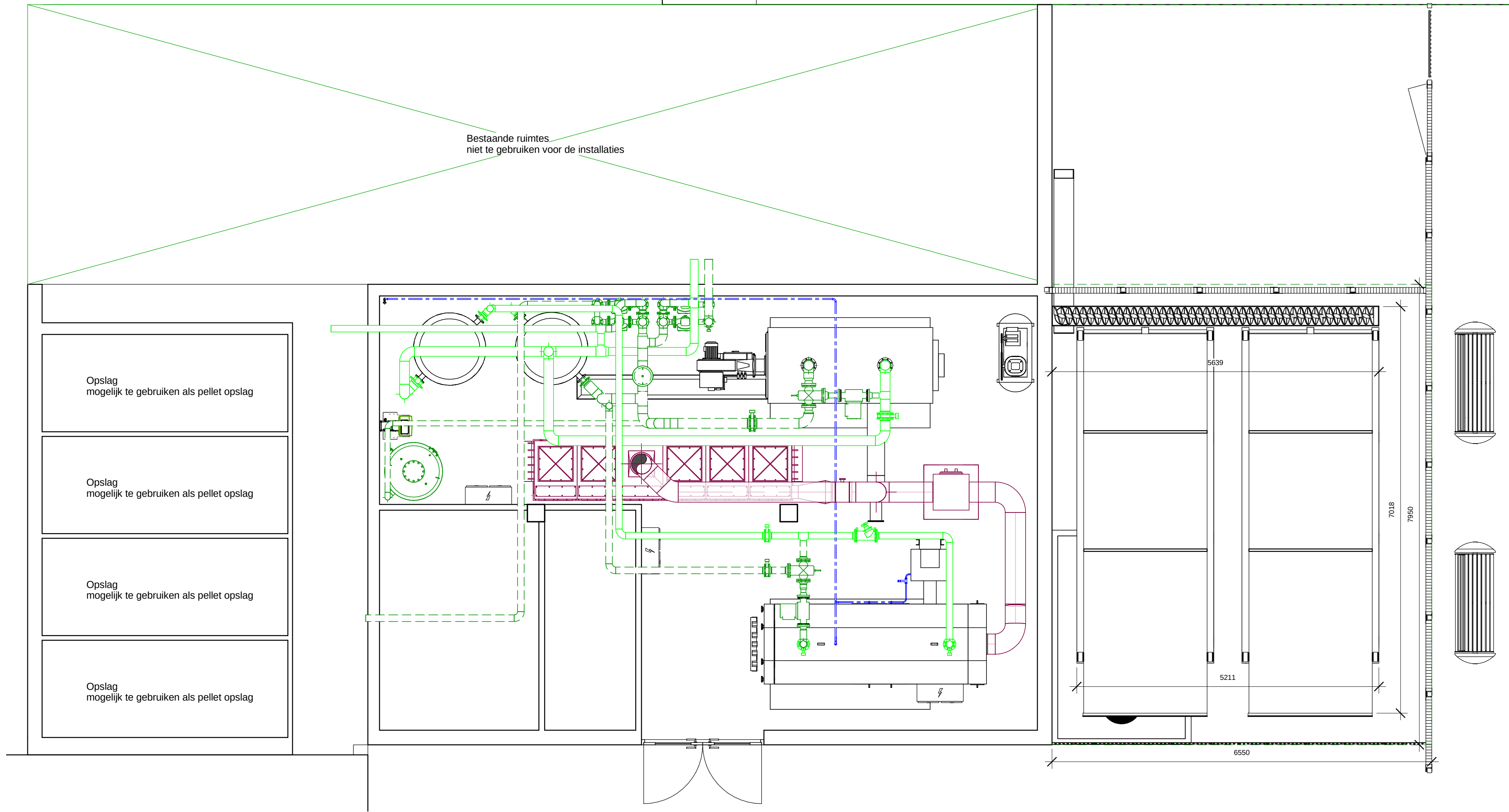
Plattegrond 1 : 50
