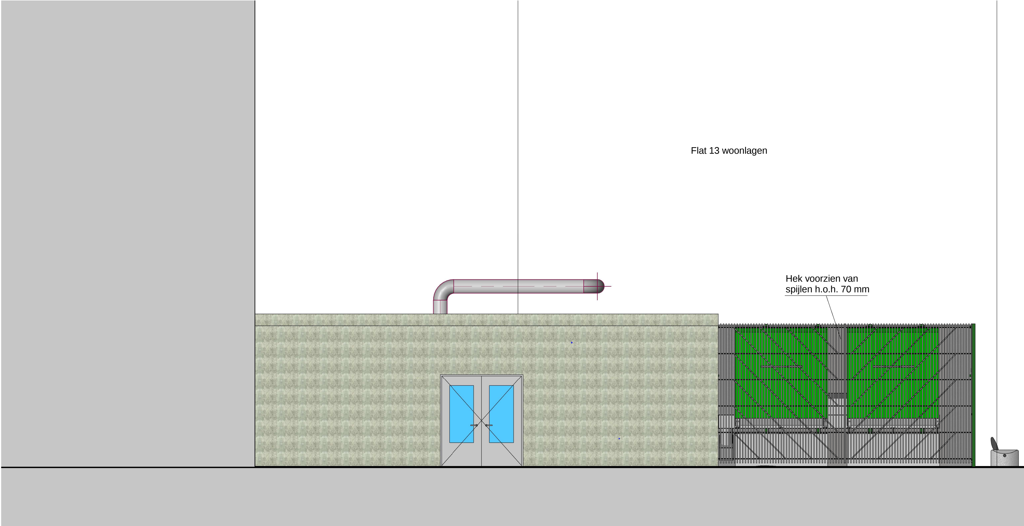
Gevelaanzicht toegang techniekruimte 1 : 50
