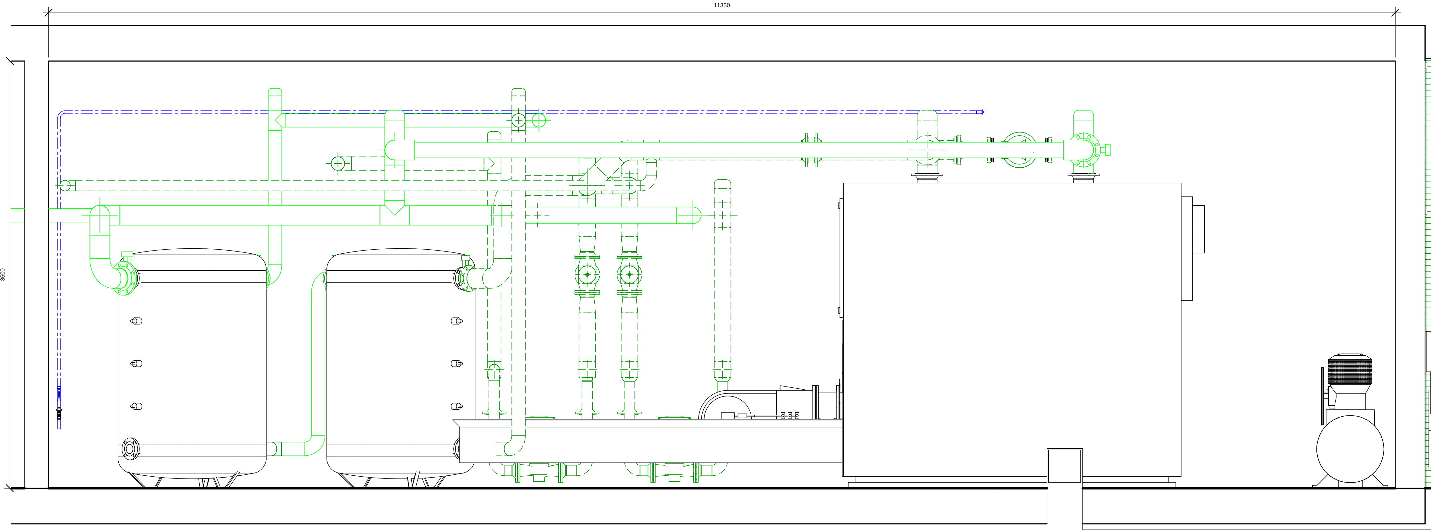
Doorsnede A-A 1 : 20
