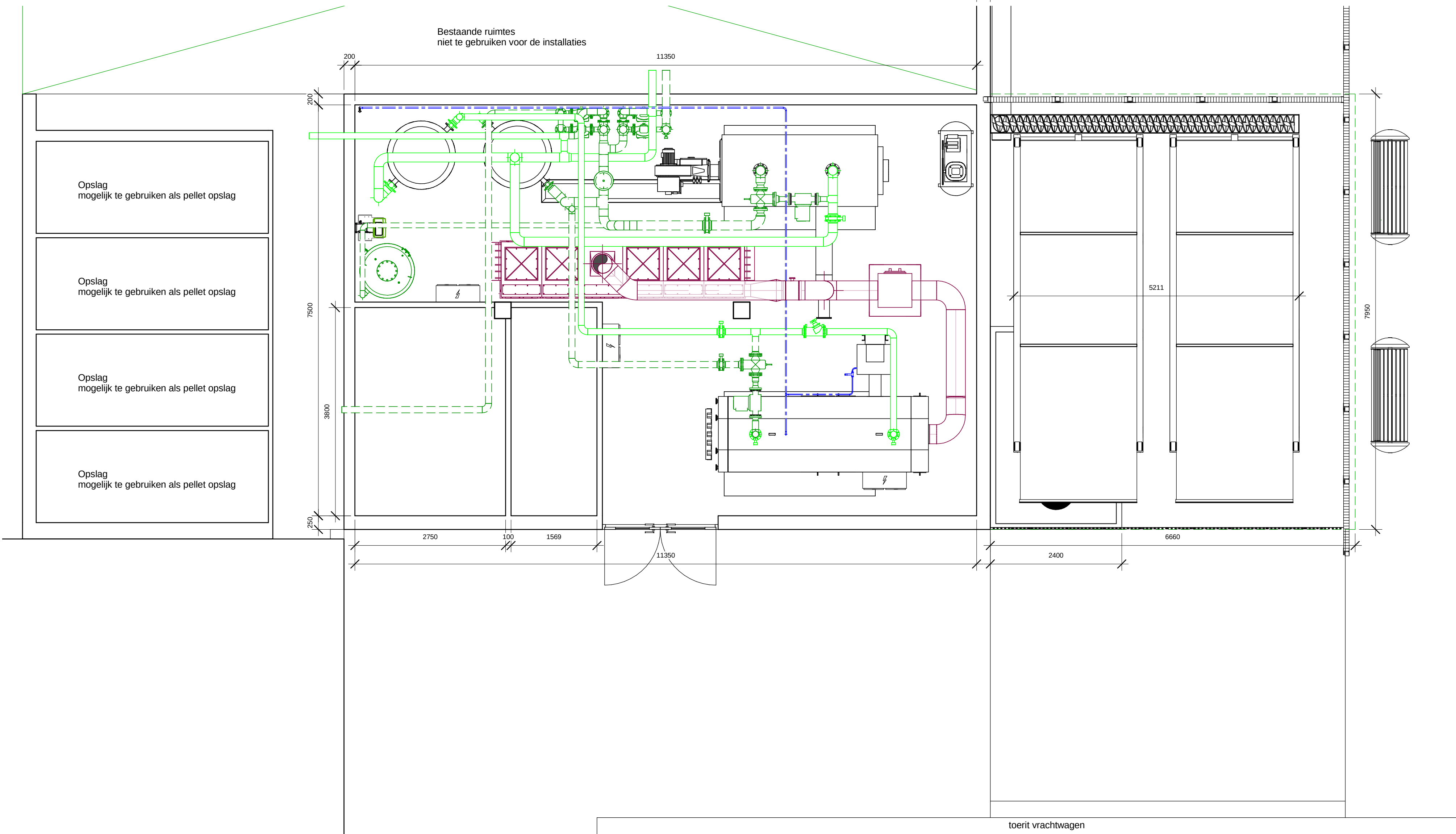
Plattegrond 1 : 50
