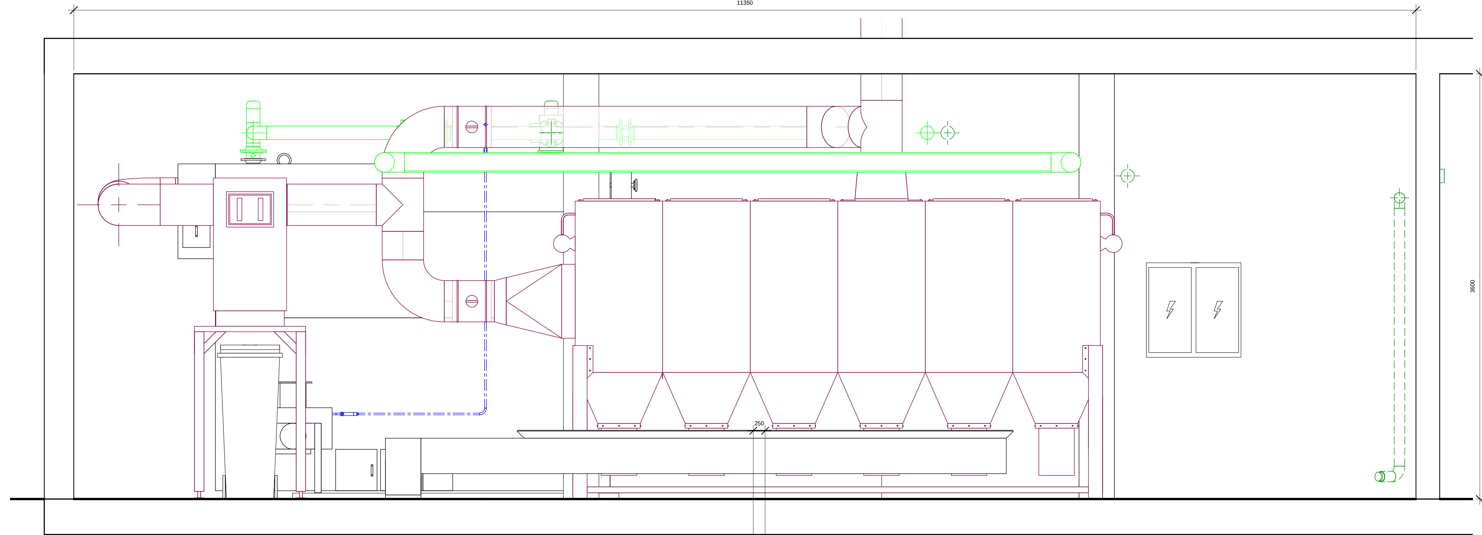
Doorsnede B-B 1 : 20
