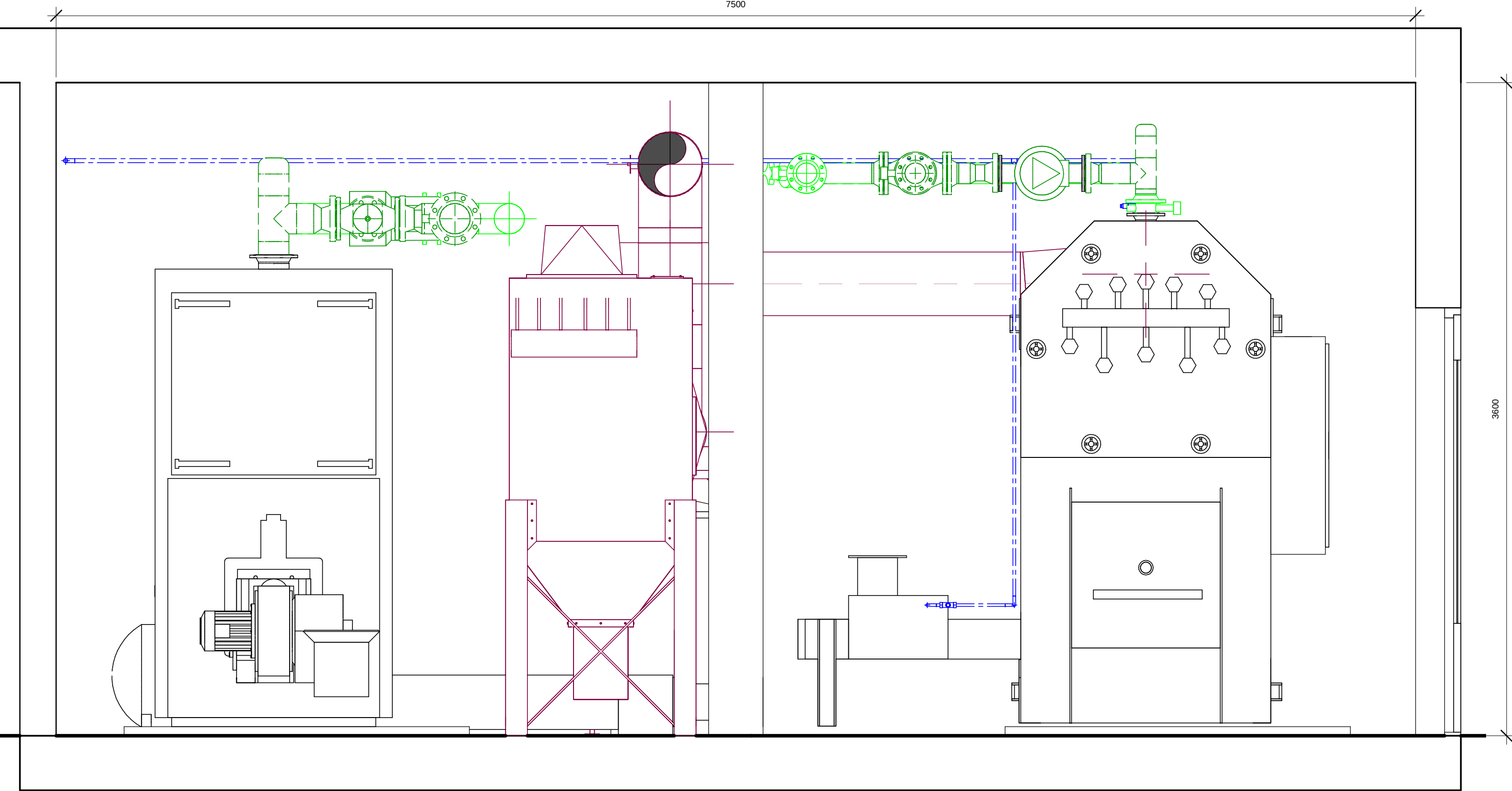
Doorsnede C-C 1 : 20
