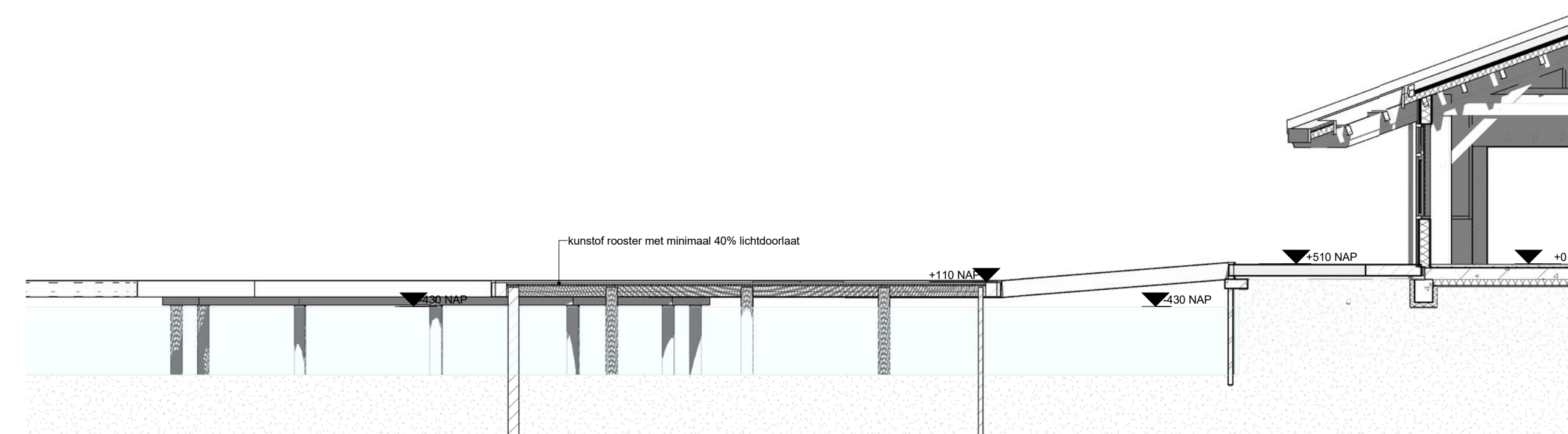
Doorsnede Vonders
