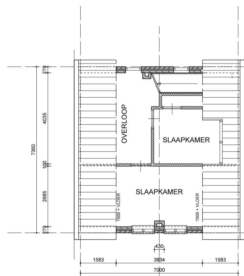
VERDIEPING BESTAAND
