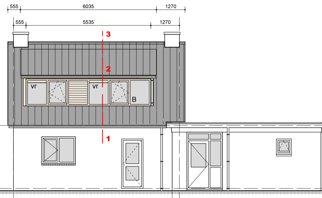
ZIJGEVEL RECHTS GEWIJZIG
