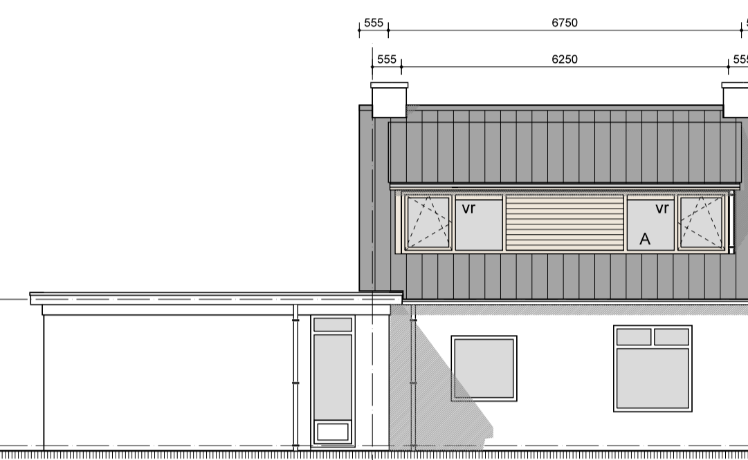
ZIJGEVEL LINKS GEWIJZIG
