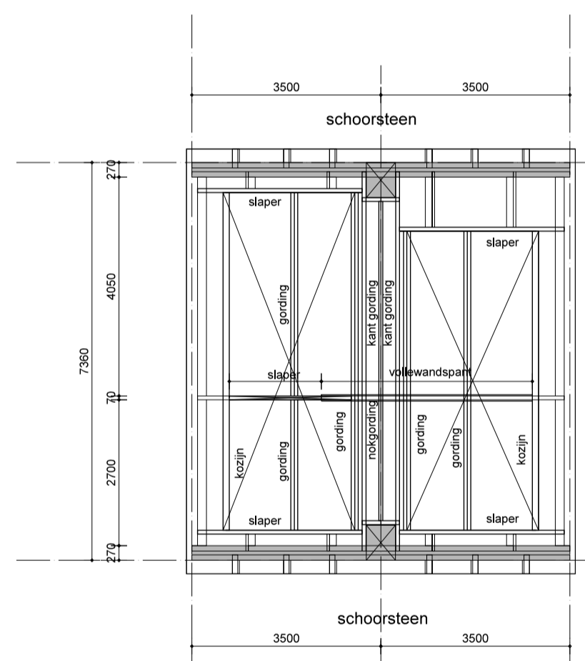
DAKCONSTRUCTIE VUREN HOUTEN GORDINGEN KAPCONSTRUCTIE bestaande gordingen 65 x 180 mm isolerende dakelementen fabr. ISOBOUW type Slimfix 3.5 3/3 Rc = 3.5 m2KW panlatten 22 x 46 mm keramische dakpannen OVH
