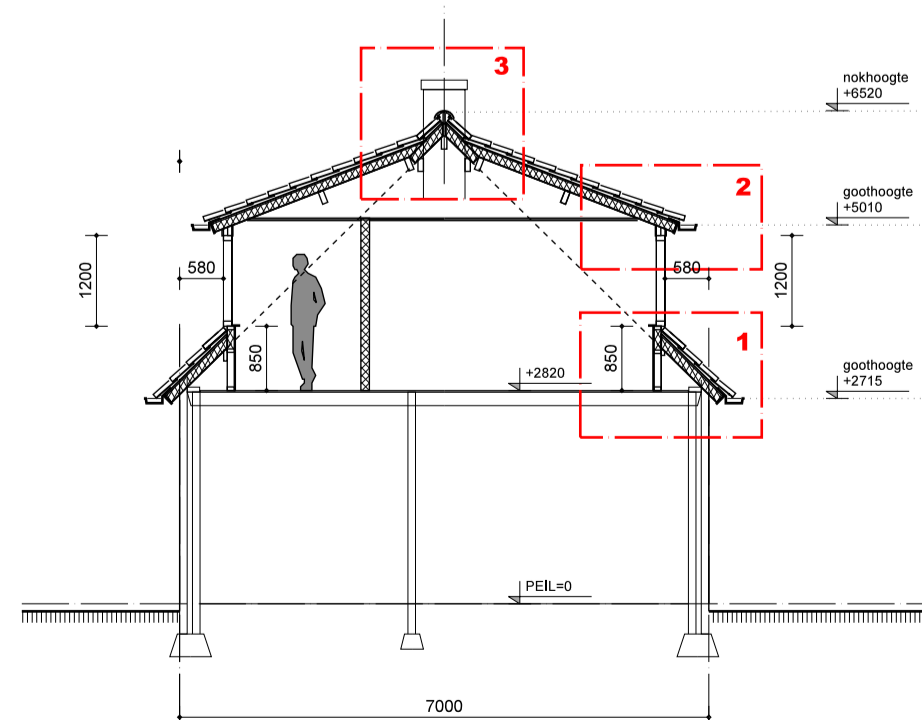
DOORSNEDE A-A GEWIJZIG
