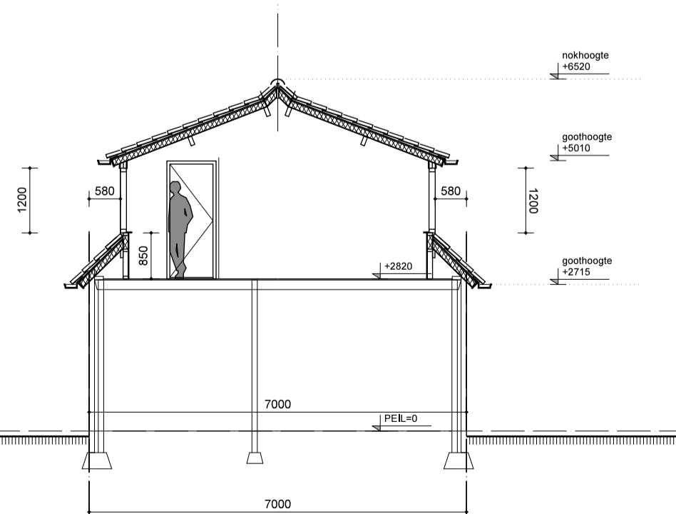
DOORSNEDE B-B GEWIJZIG
