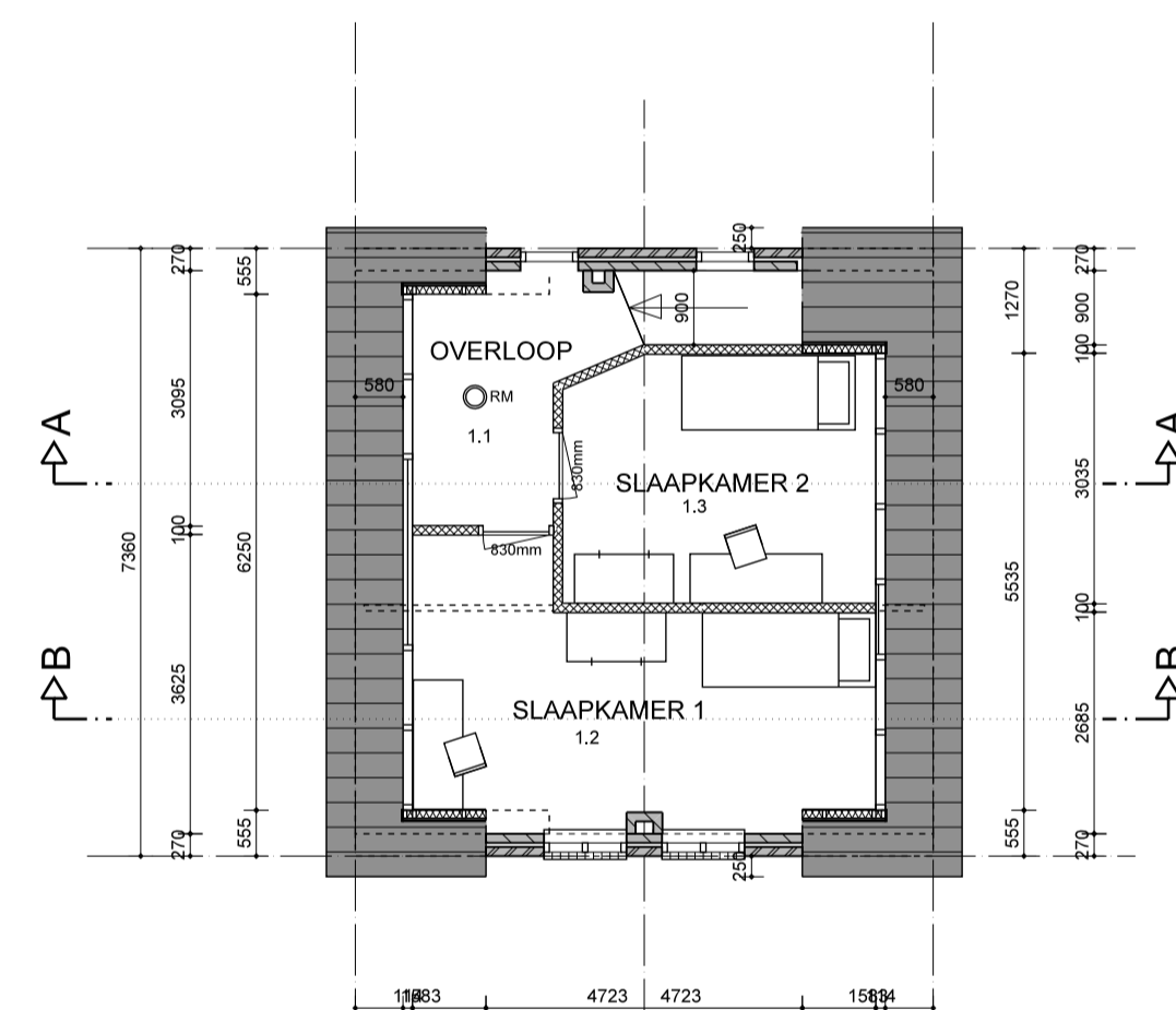
VERDIEPING GEWIJZIG
