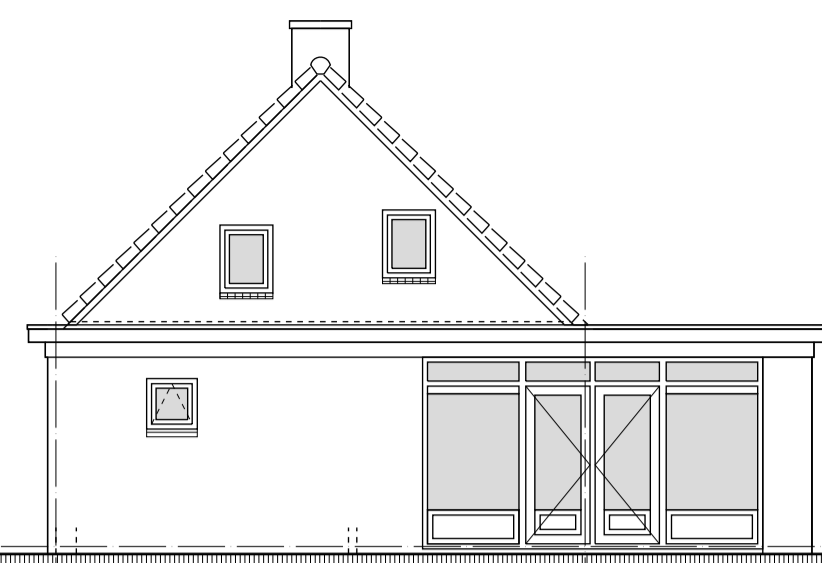
ACHTERGEVEL BESTAAND
