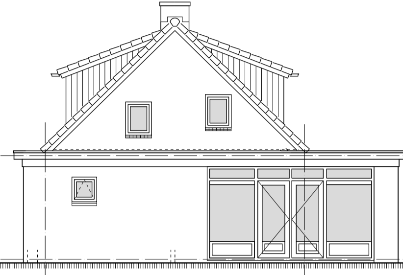
ACHTERGEVEL GEWIJZIG
