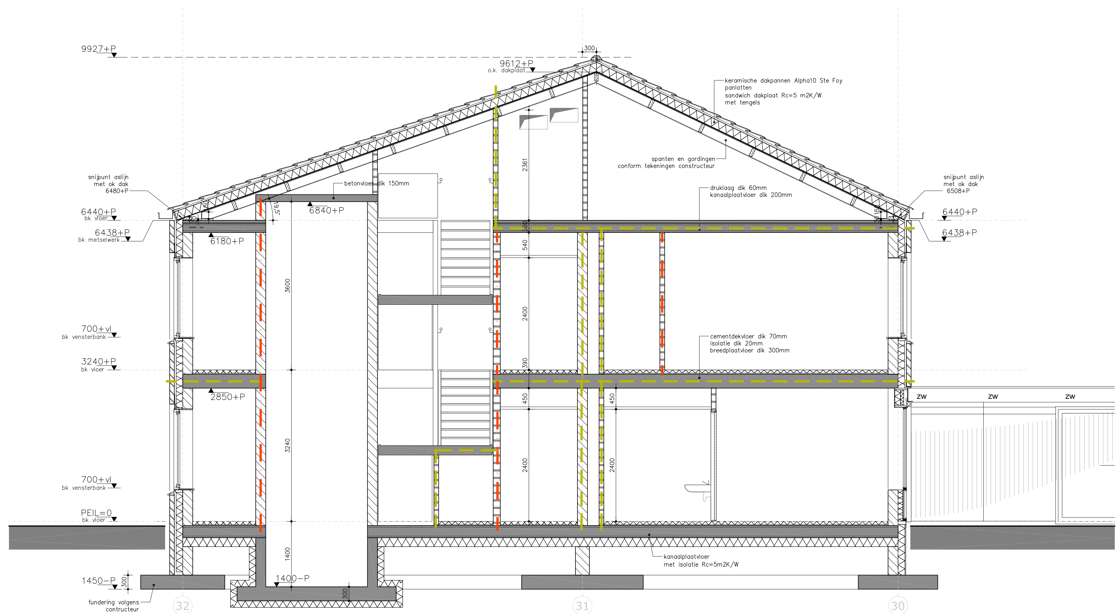
doorsnede B3
