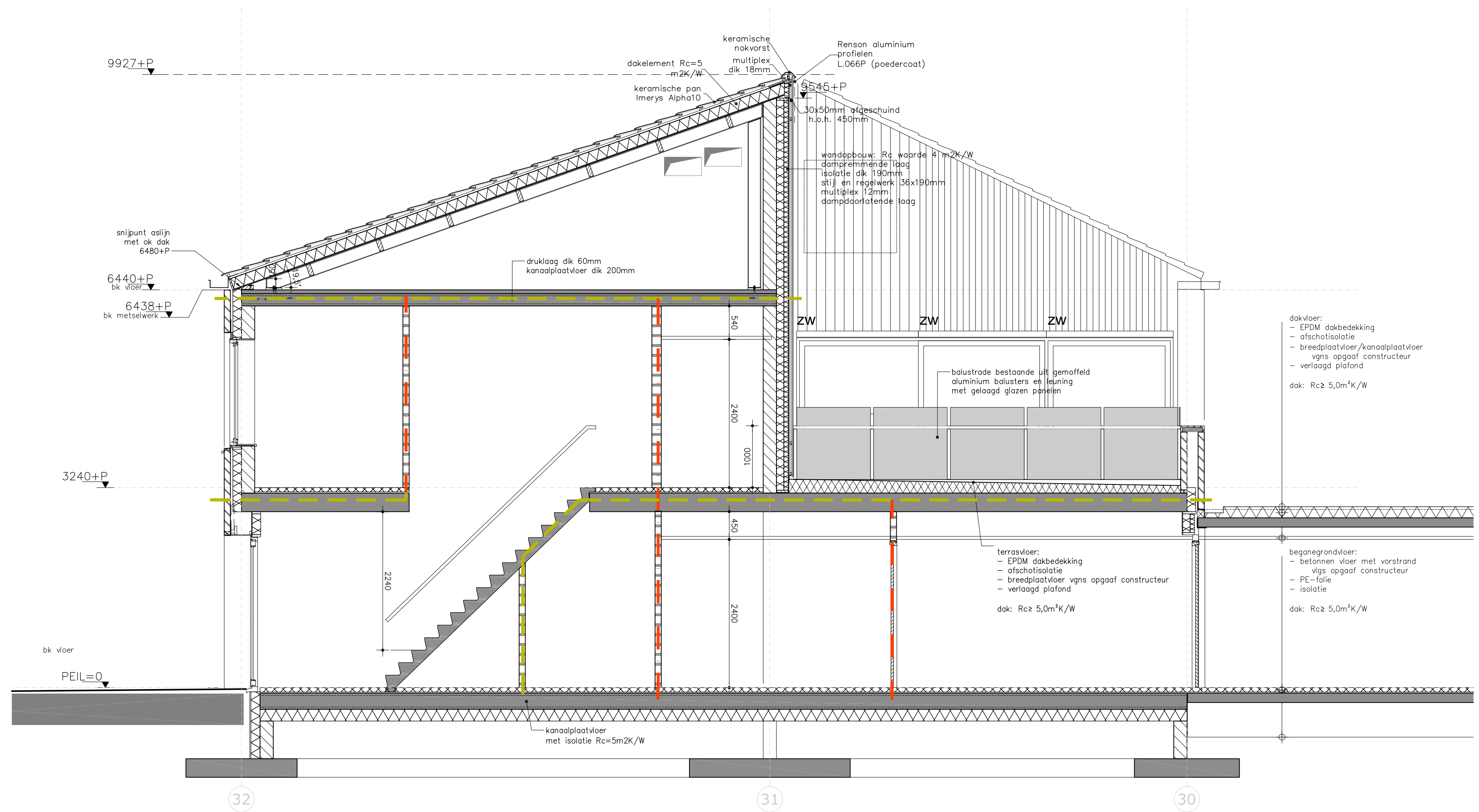
doorsnede A3
