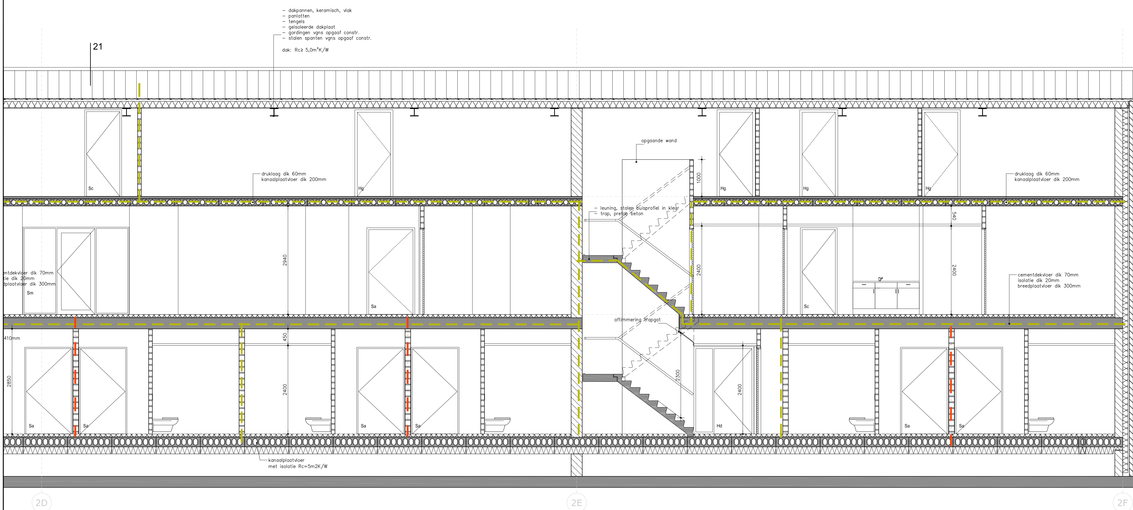
doorsnede C-2
