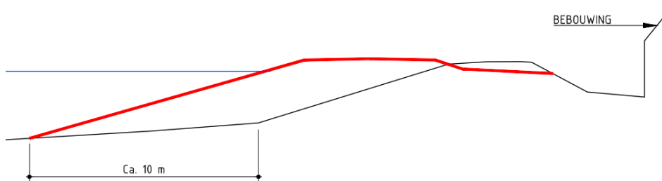
Figuur 7.3: Dwarsprofiel dijkvak 50.530.16
