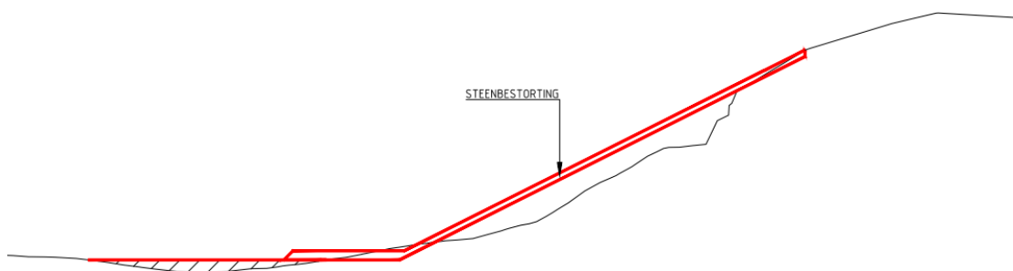
Figuur 5.6: Principe dwarsprofiel voor het verflauwen van de oevers
