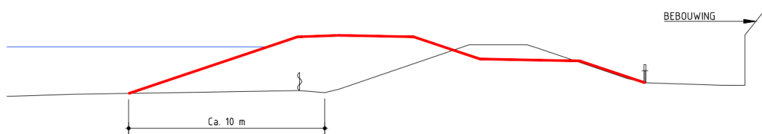
Figuur 4.5: Dwarsprofiel dijkvak 50.410.10
