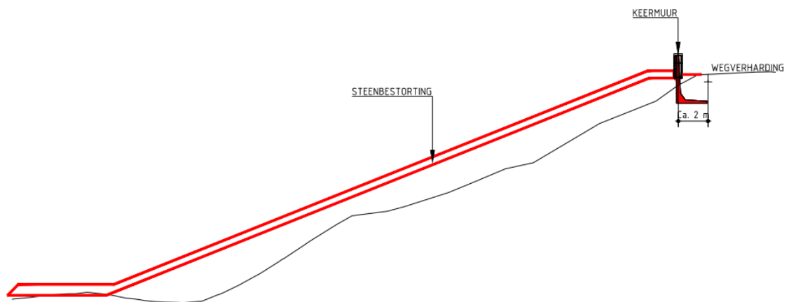
Figuur 4.9: Dwarsprofiel dijkvak 50.410.14
