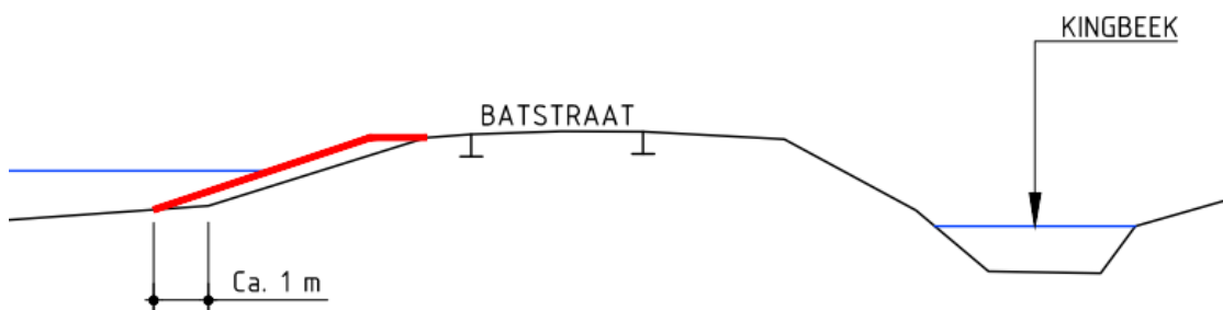
Figuur 5.8: Dwarsprofiel dijkvak 50.510.12
