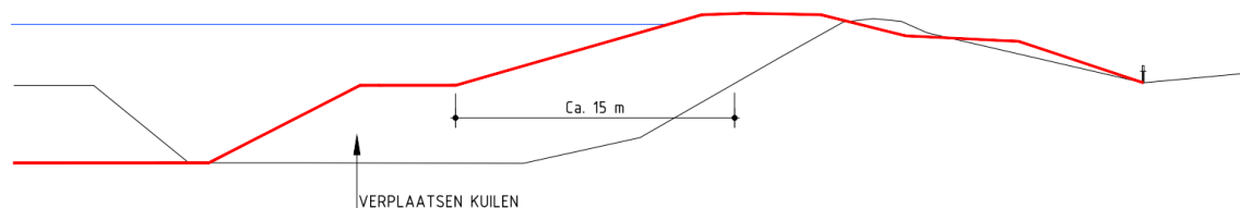
Figuur 9.3: Dwarsprofiel dijkvak 50.550.2
