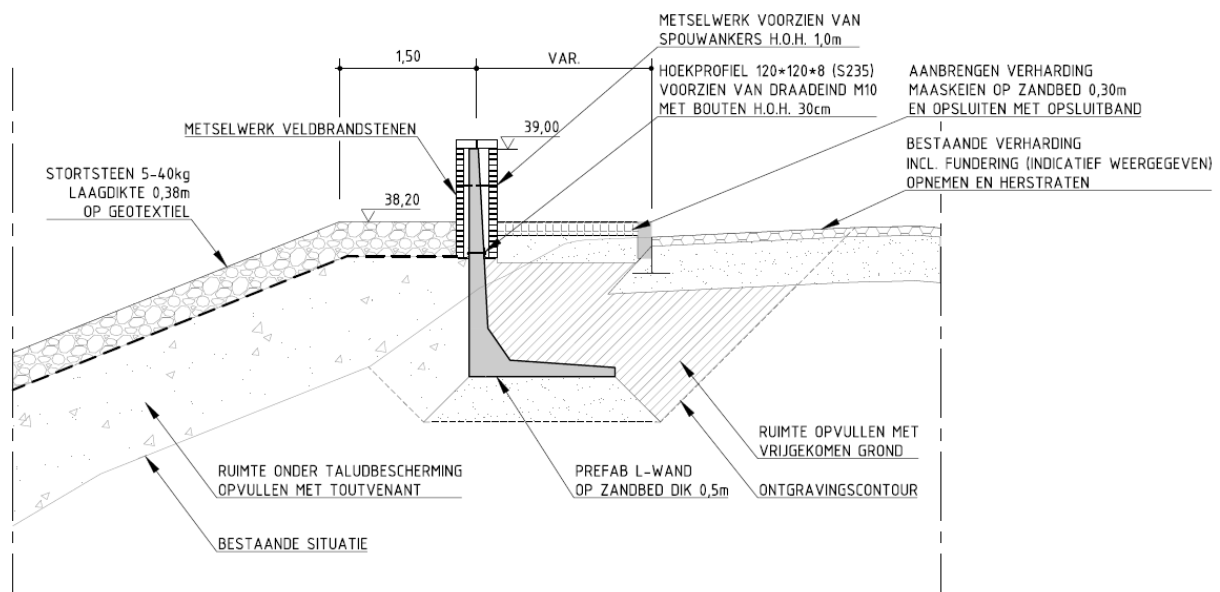
PRINCIPEDOORSNEDE 2 KEERWAND MET STOEP
