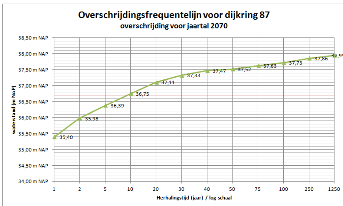
Afbeelding 3.2 Overschrijdingsgrafiek 2070
