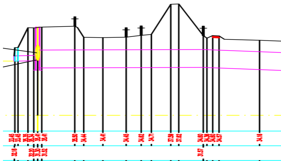
Afbeelding 2.3 WBL leiding DN1700 met de kering (grootste ophoging)
