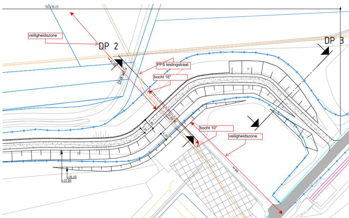
Afbeelding 2.1 Bovenaanzicht parallelle ligging leidingen aan de kade
