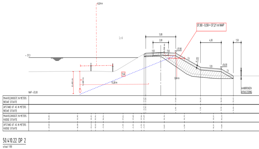
Afbeelding 4.1 bepaling afslag profiel bij breuk leiding
