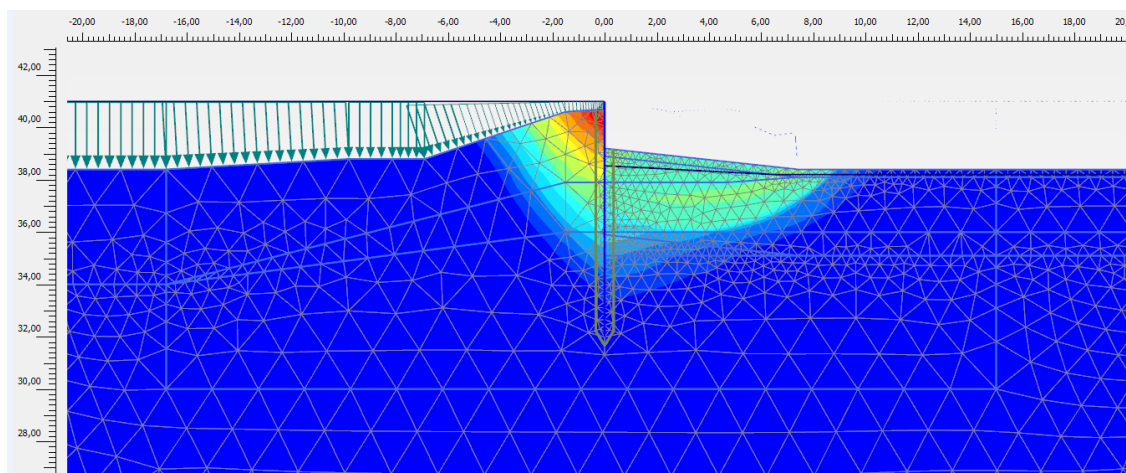
Figuur 5.1: Bezwijkmechanisme damwand-berekening
