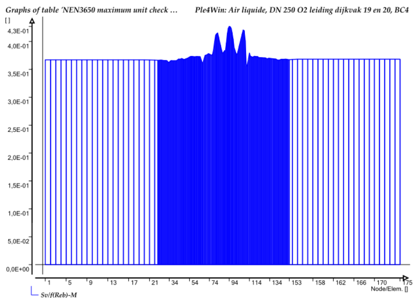
Afbeelding 4.3 Berekende toetsspanningen van de maatgevende DN250leiding in dijkvak 19 en 20, BC 4
