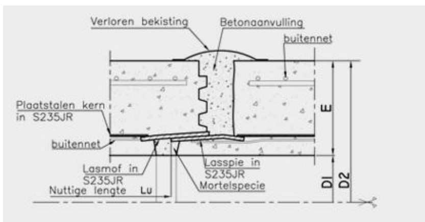
Abbeelding 2.1 Principe schets van een voeg van een betonleiding met plaatstalenkern
