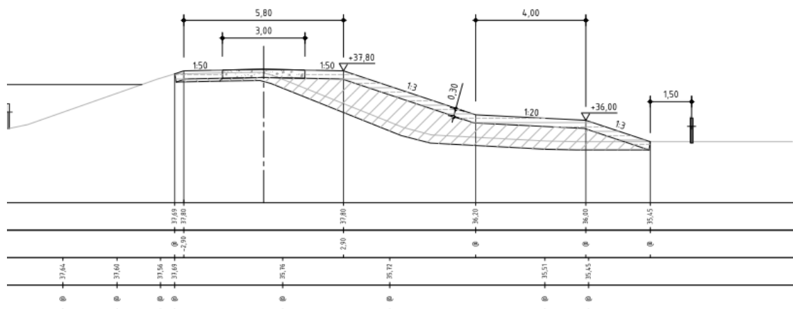
Afbeelding 2.2 Dwarsdoorsnede kade
