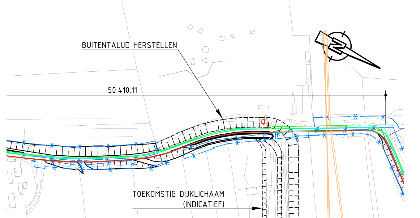
INDICATIE AANSLUITING TOEKOMSTIG DIJKLICHAAM SCHAAL 1:2000
