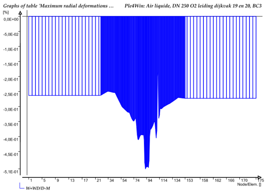
Afbeelding 4.4 Berekende deflectie van de maatgevende DN250leiding in dijkvak 19 en 20, BC 3
