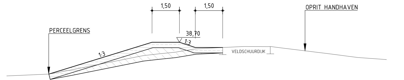
PRINCIPE DP A schaal 1:100
