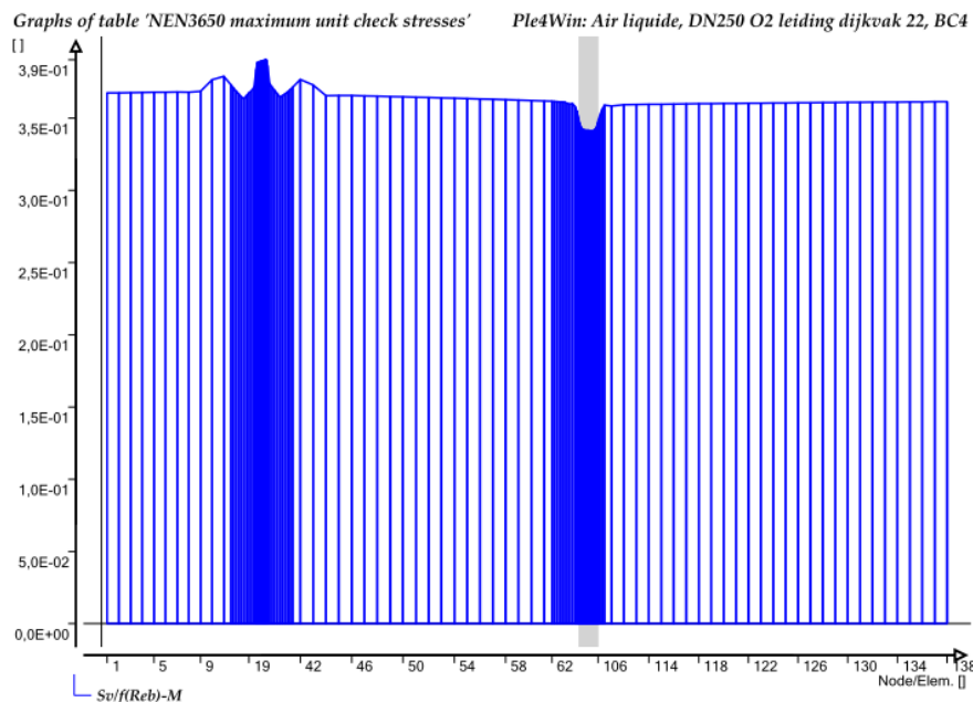
Afbeelding 4.1 Berekende toetsspanningen van de maatgevende DN250 leiding in dijkvak 22, BC 4
