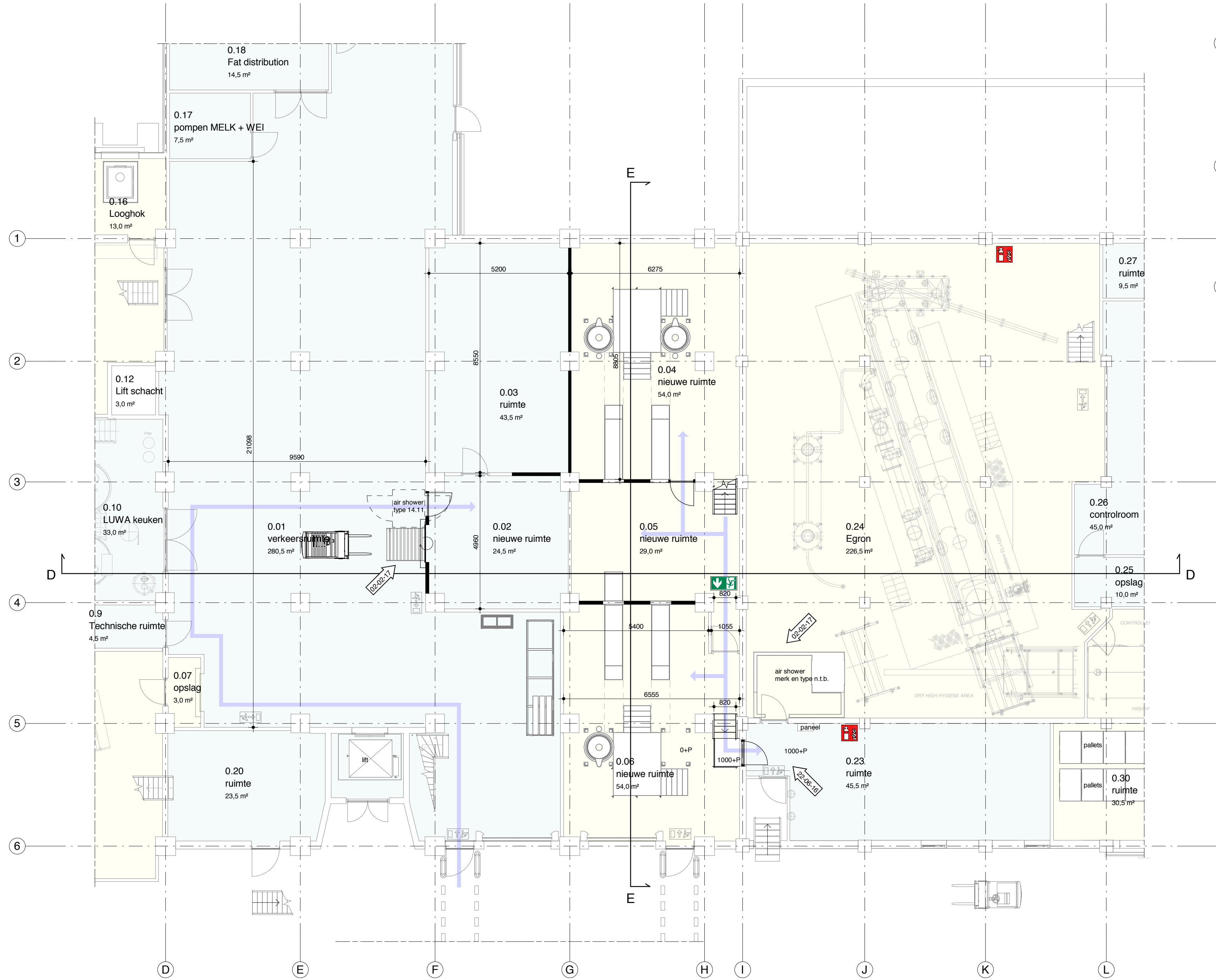
nieuwbouw begane grondvloer Luwa - Niro 0+
