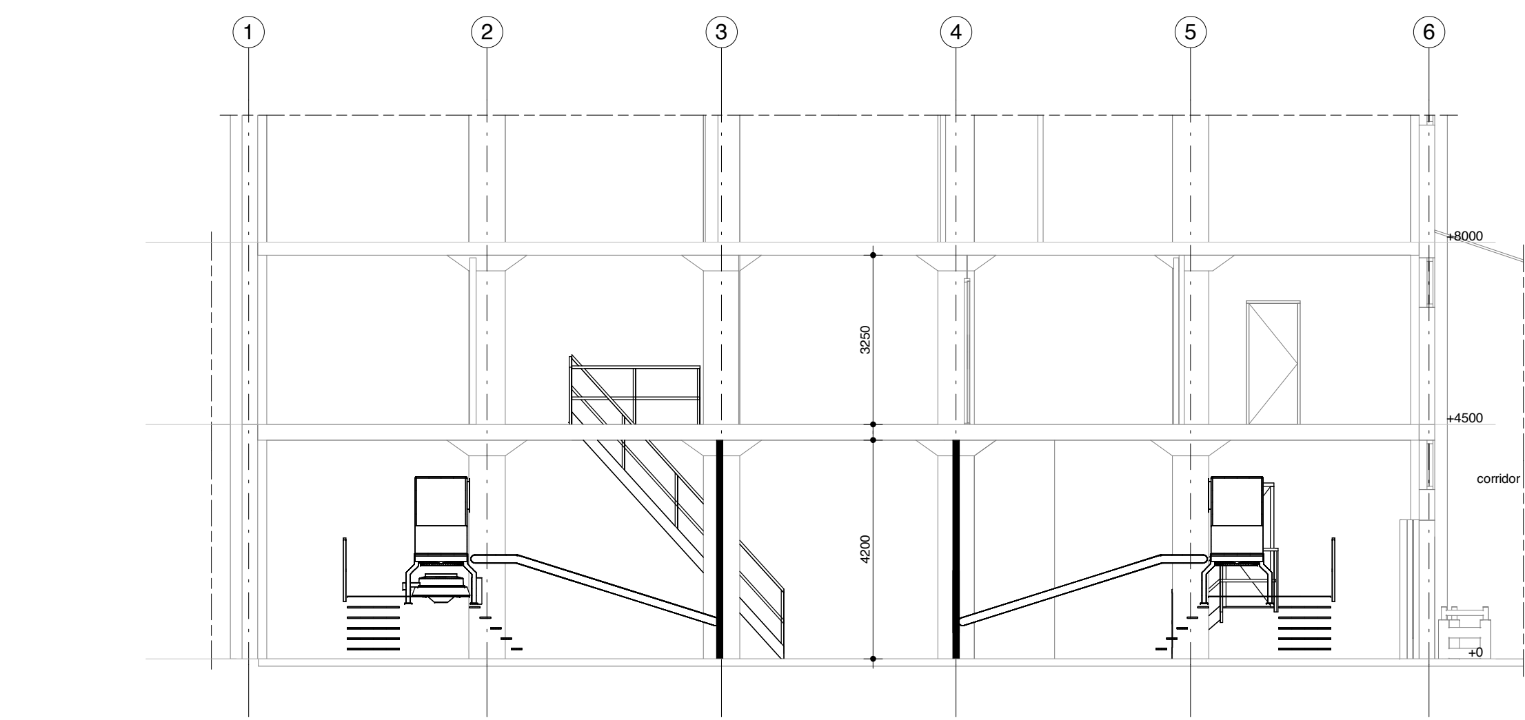
nieuwbouw doorsnede E - E
