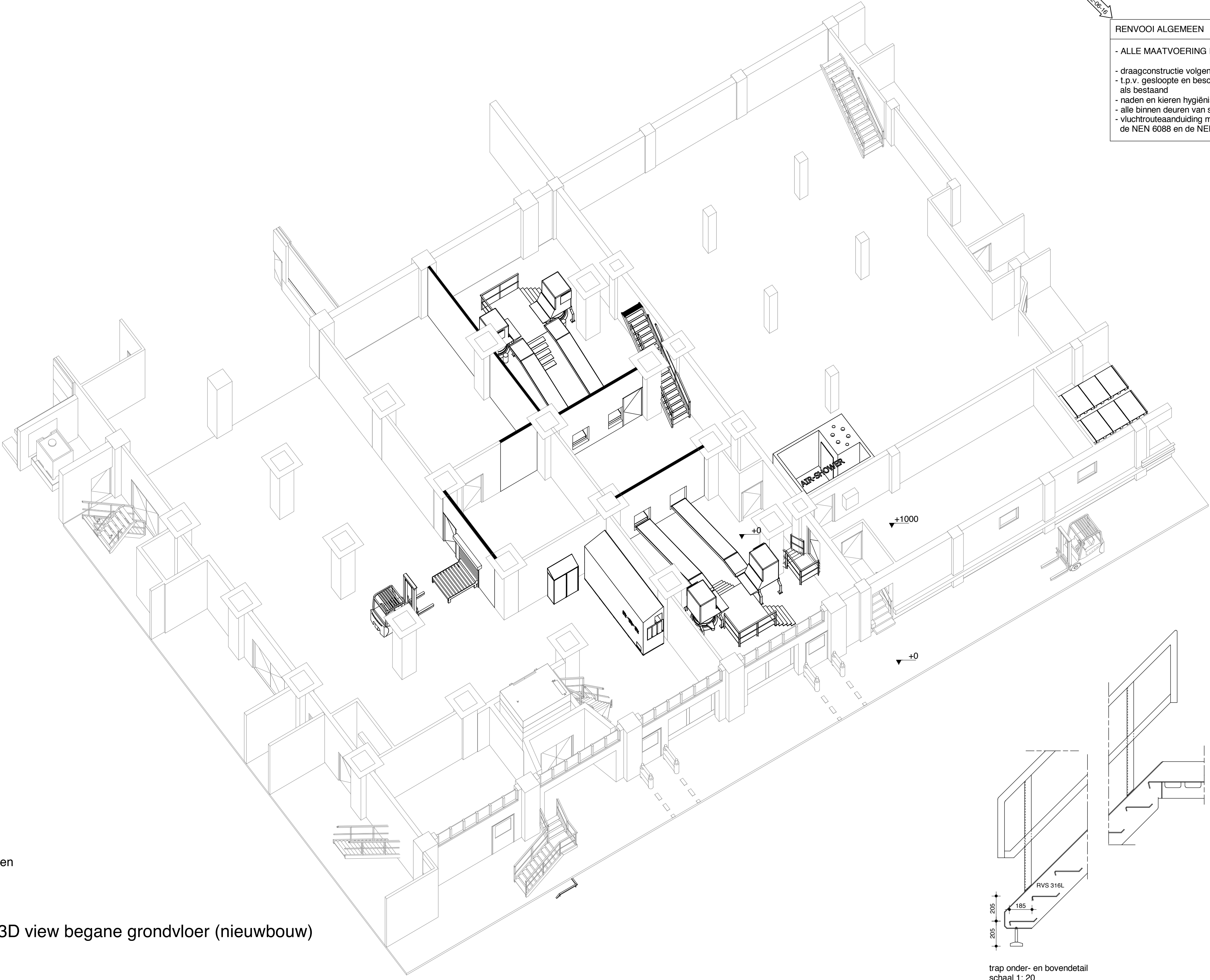
nieuwbouw begane grondvloer Luwa - Niro 0+
