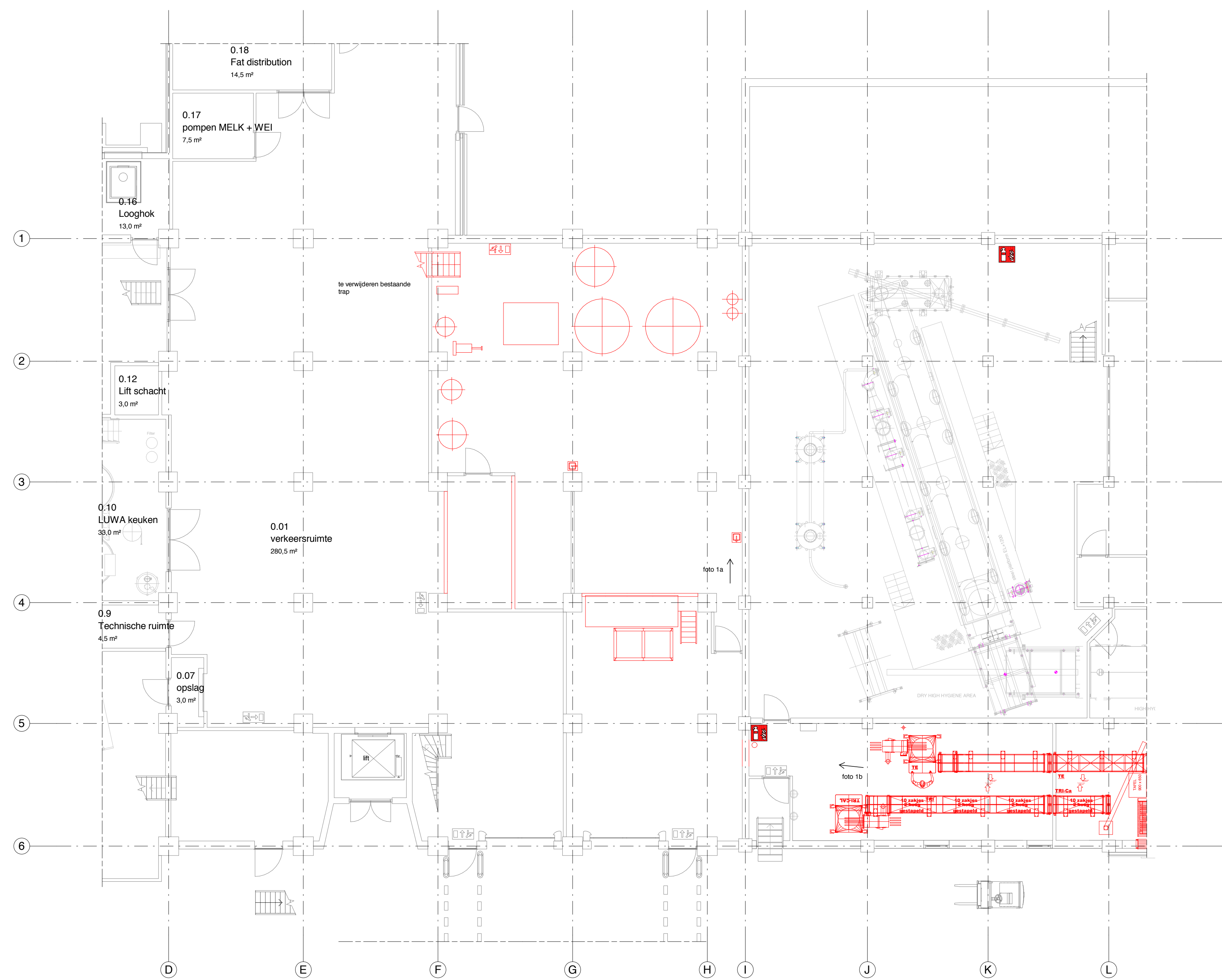
bestaand begane grondvloer Luwa - Niro 0+
