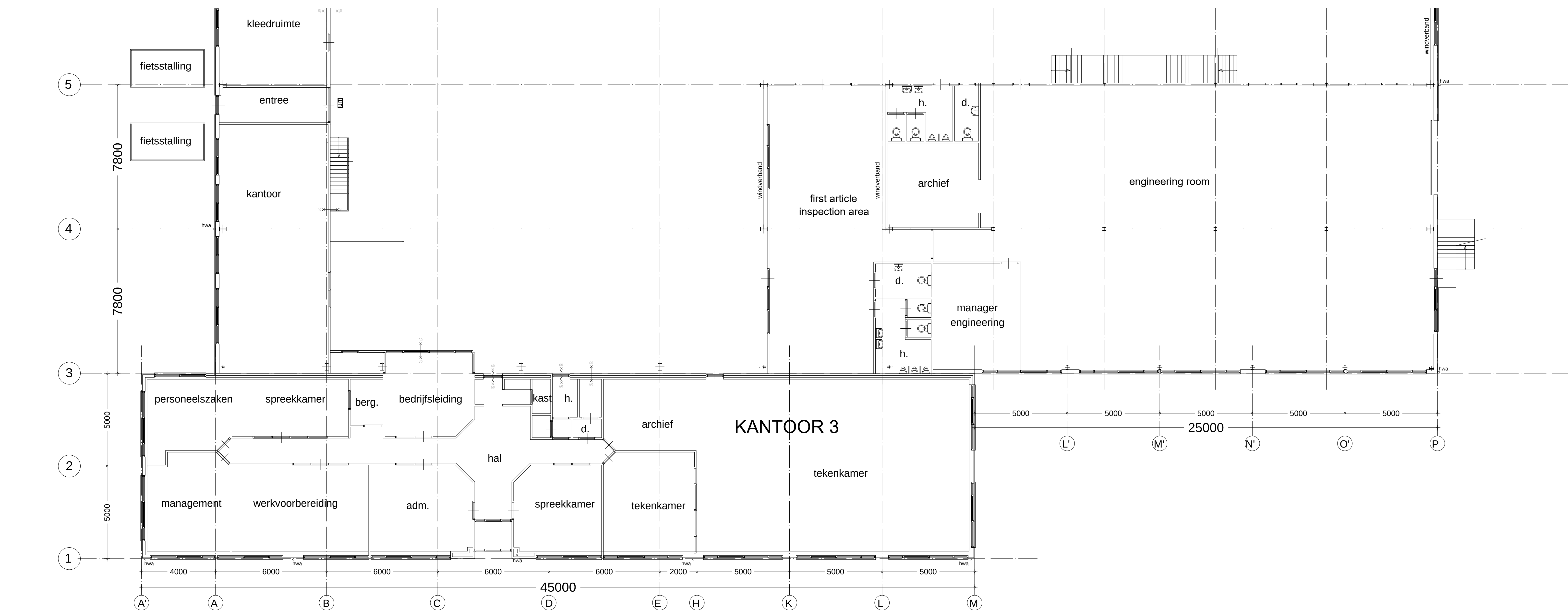
BEGANEGROND (schaal 1:100) b.k. vloer = Peil = 0
