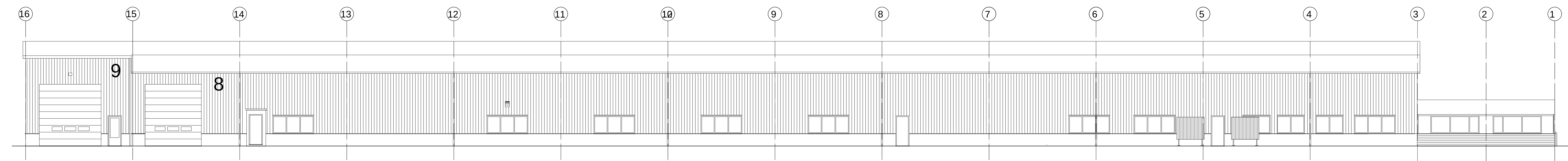
ZIJGEVEL NOORDZIJDE
