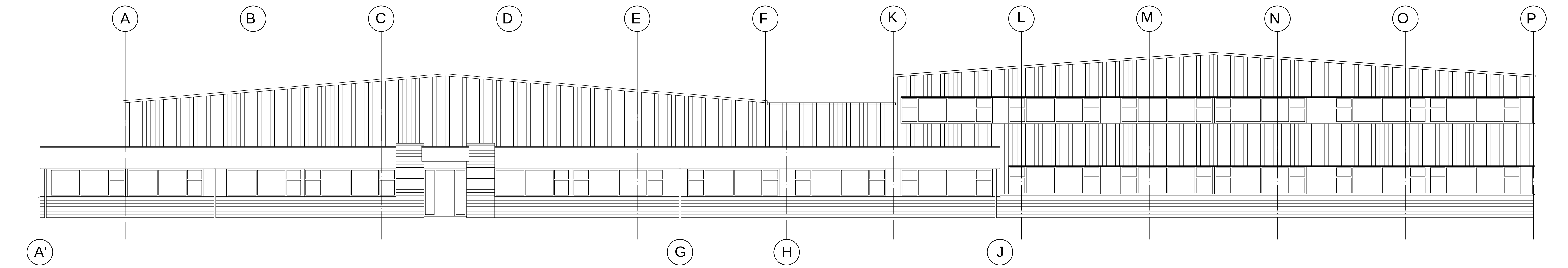
VOORGEVEL WESTZIJDE
