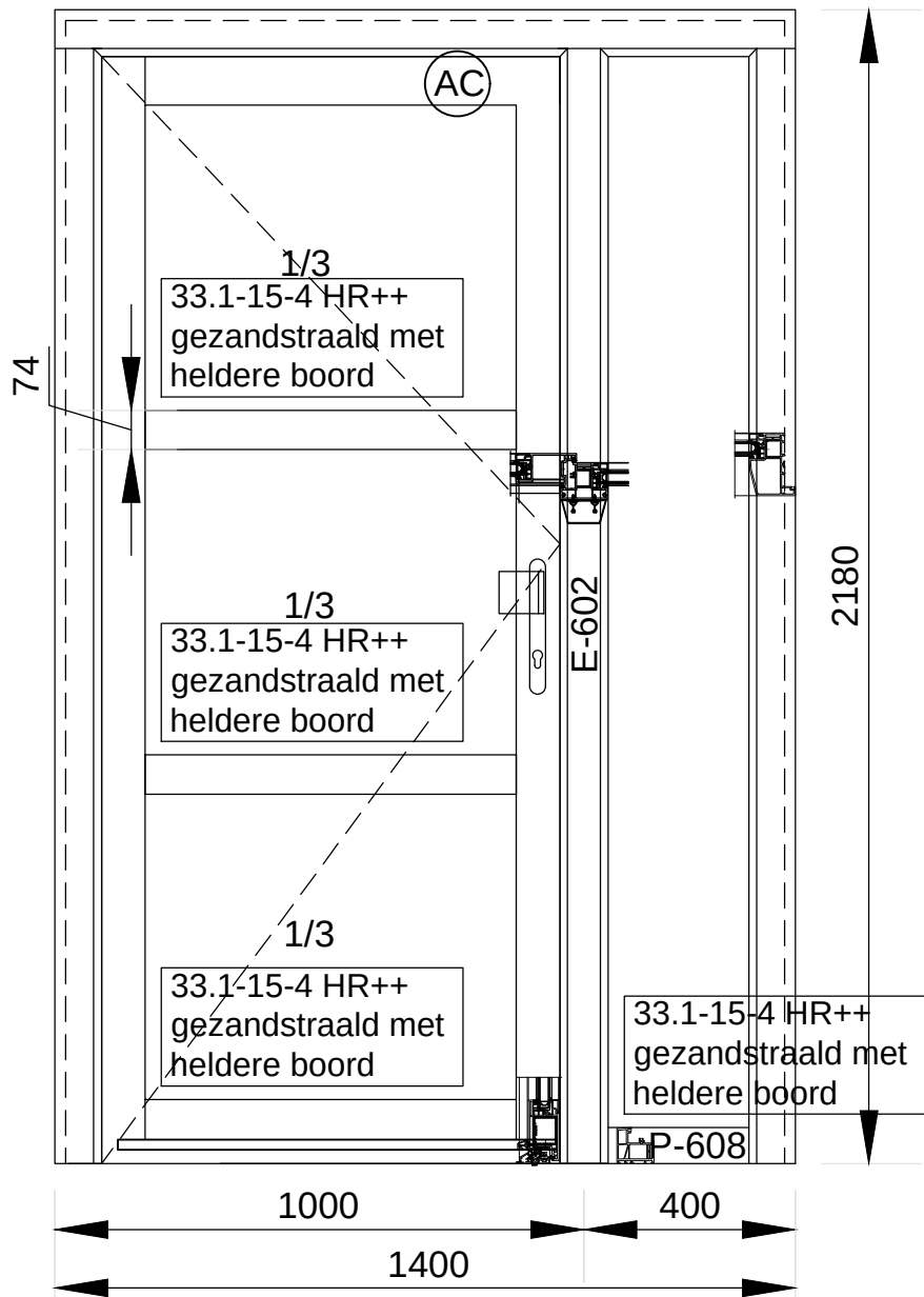
Pos 1.4 ( binnendraaiend )
