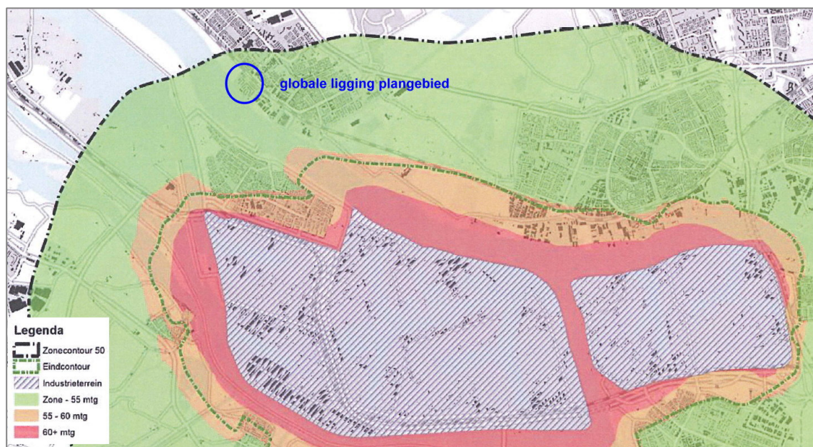
Figuur 4.2. geluidcontouren industrieterrein Botlek-Pernis
