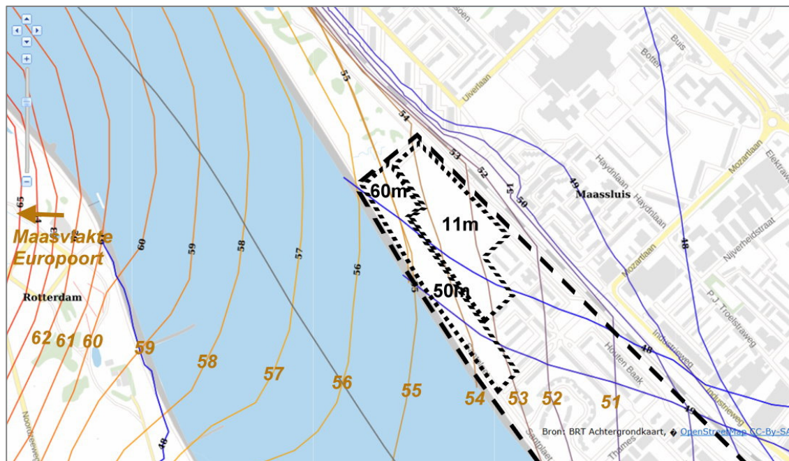
Figuur 4.5. contourenkaart van industrierrein Maasvlakte-Europoort
