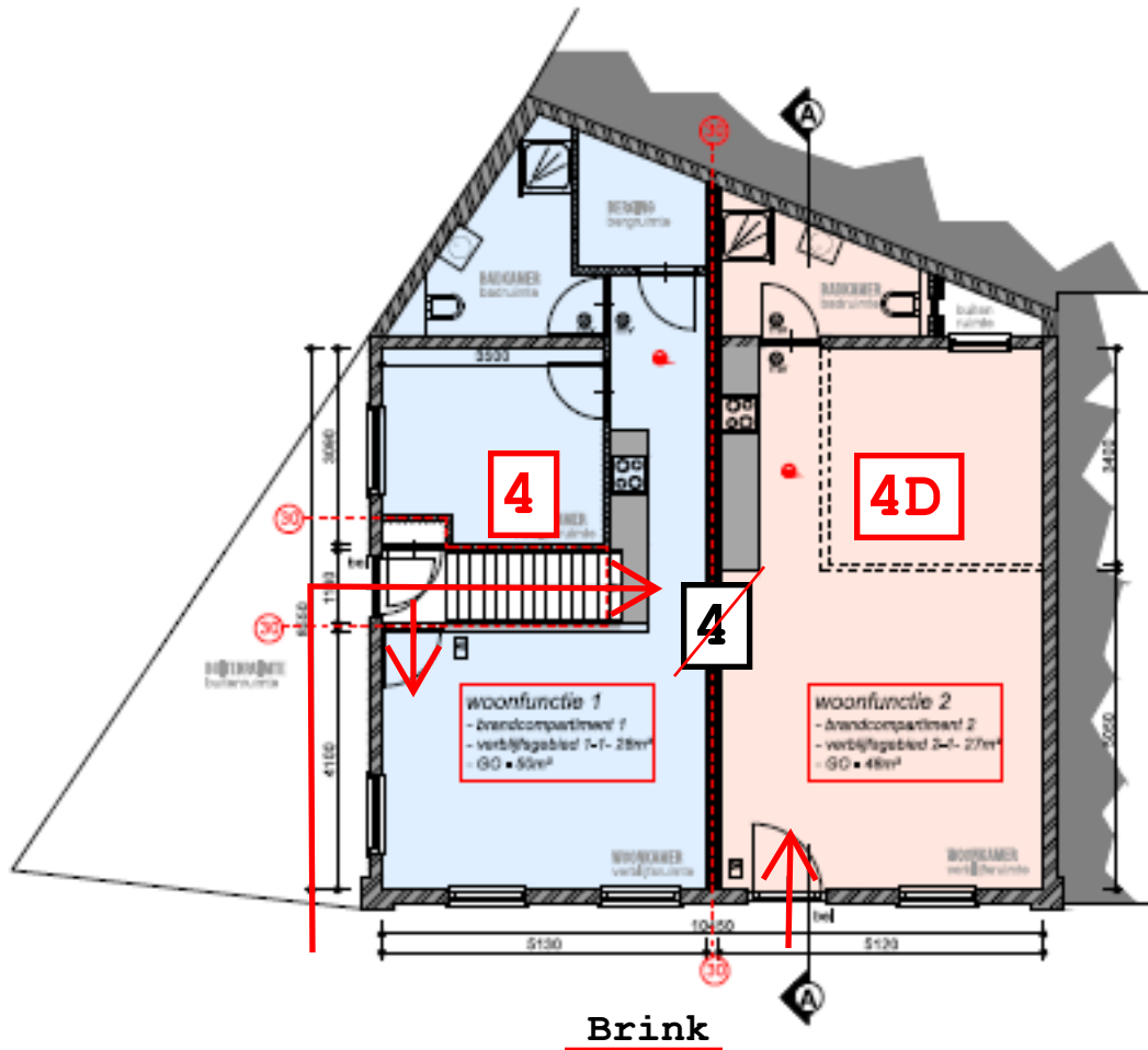
BEGANE GROND NIUWE SITUATIE
