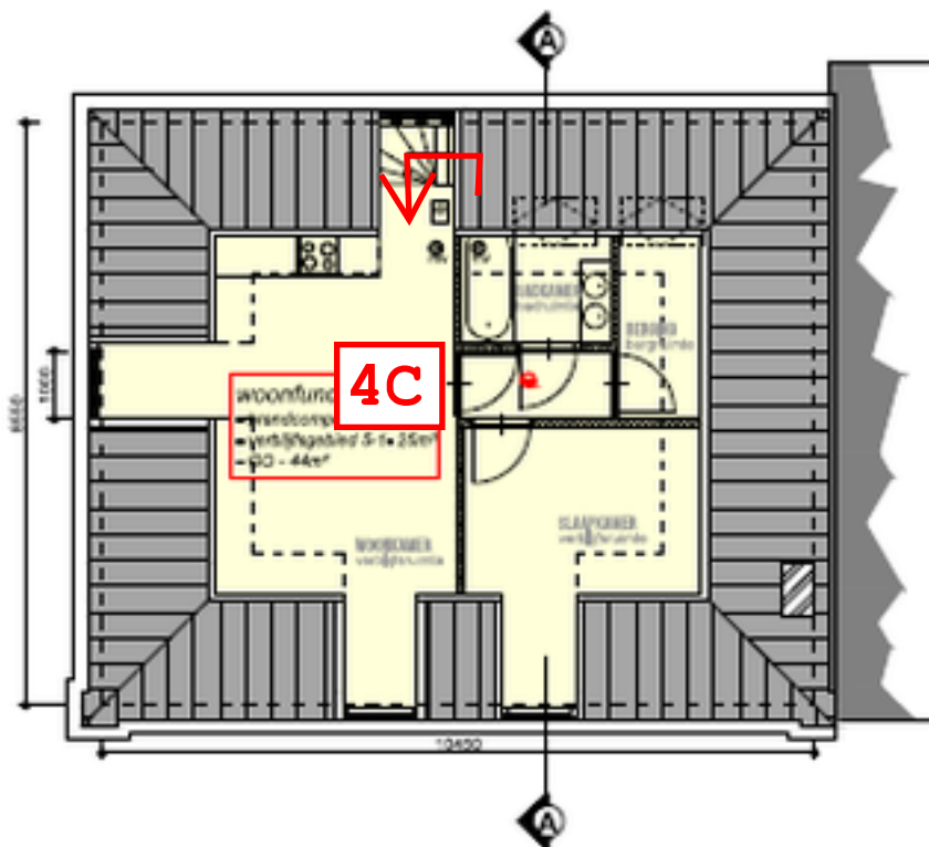
TWEDE VERDIEPING NIUWE SITUATIE
