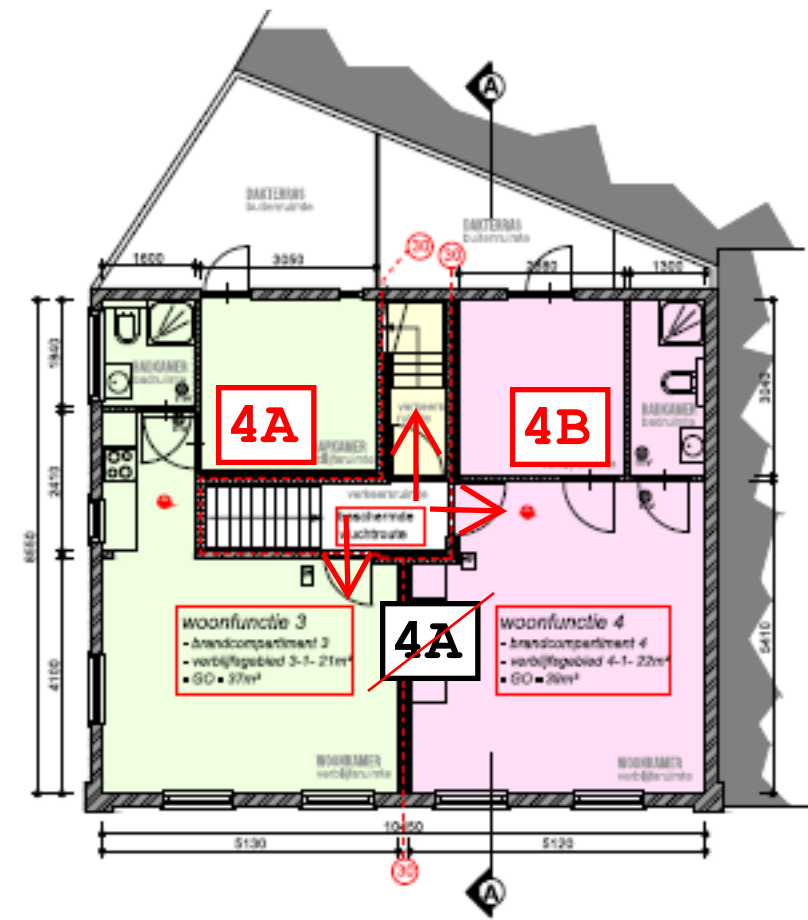
EERSTE VERDIEPING NIUWE SITUATIE
