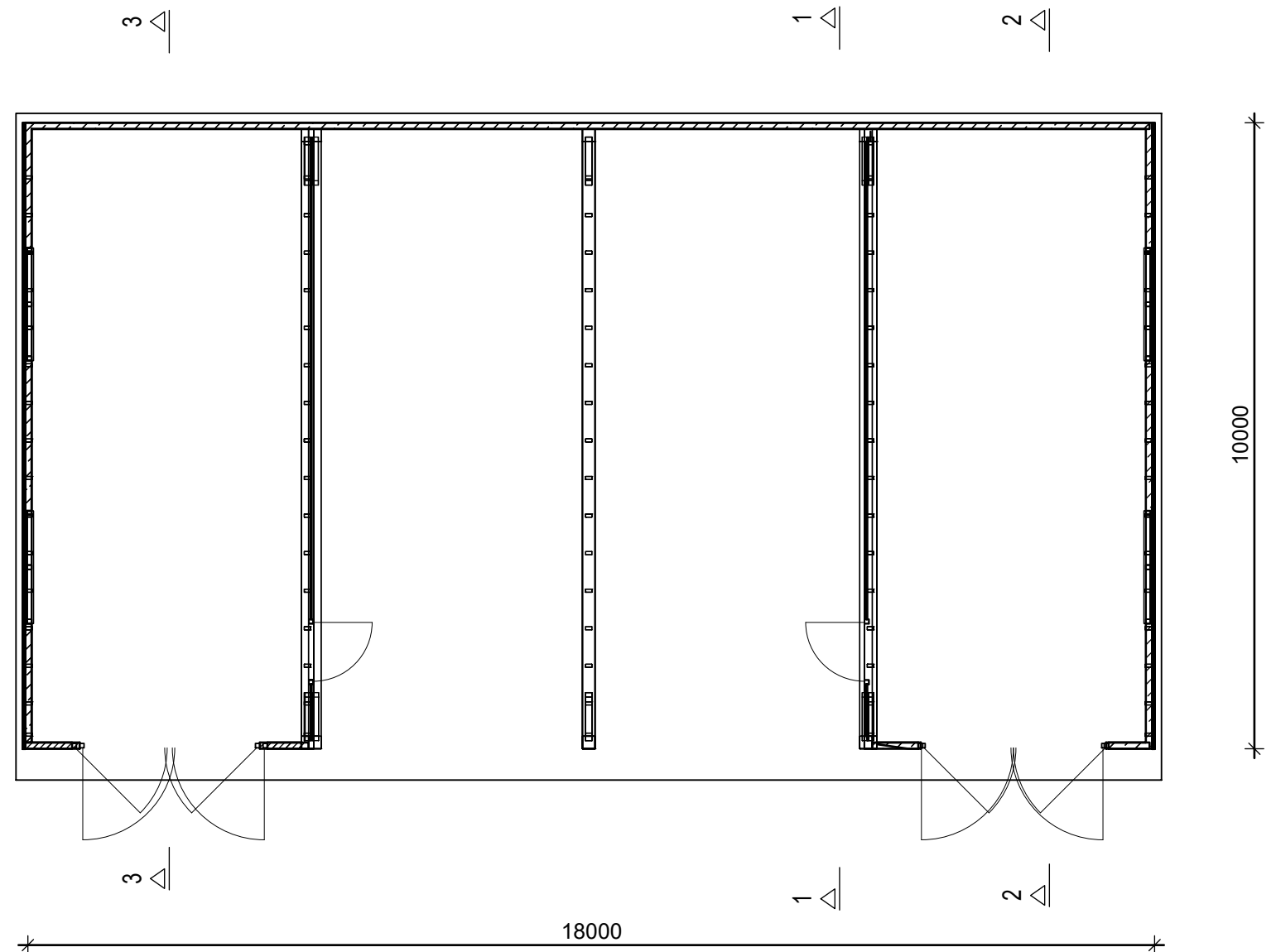
Platte grond
