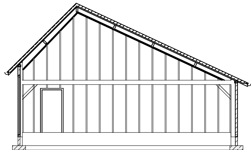
doorsnede 2 - 2
