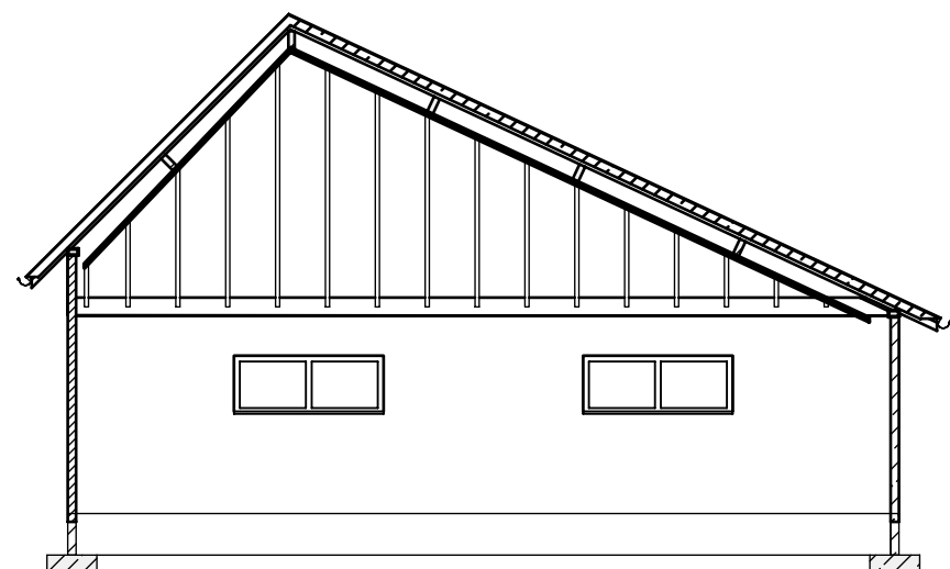
doorsnede 3 - 3
