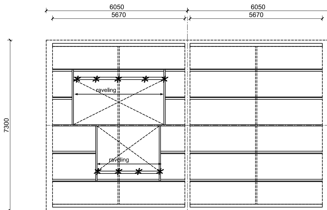
KAPPLAN (nieuw)
