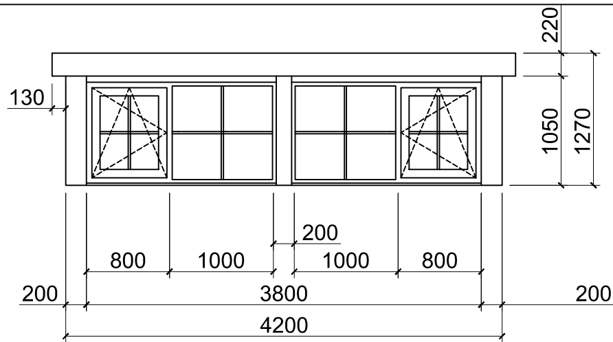
AANZICHT DAKKAPEL ACHTERGEVEL (schaal 1:50)
