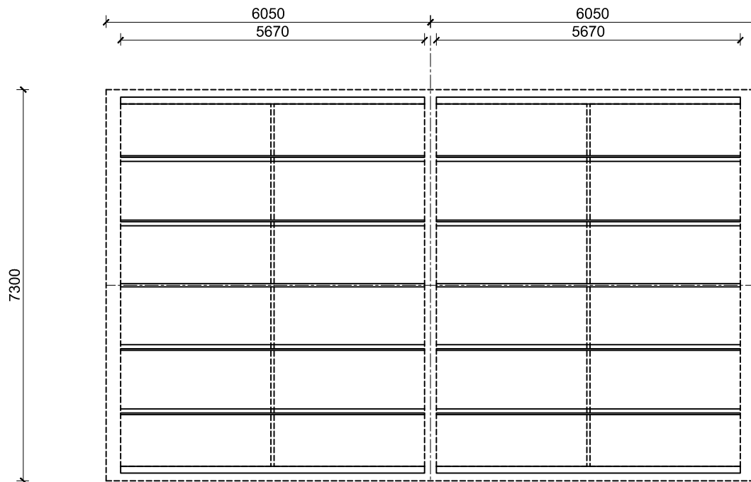
KAPPLAN (bestaand)
