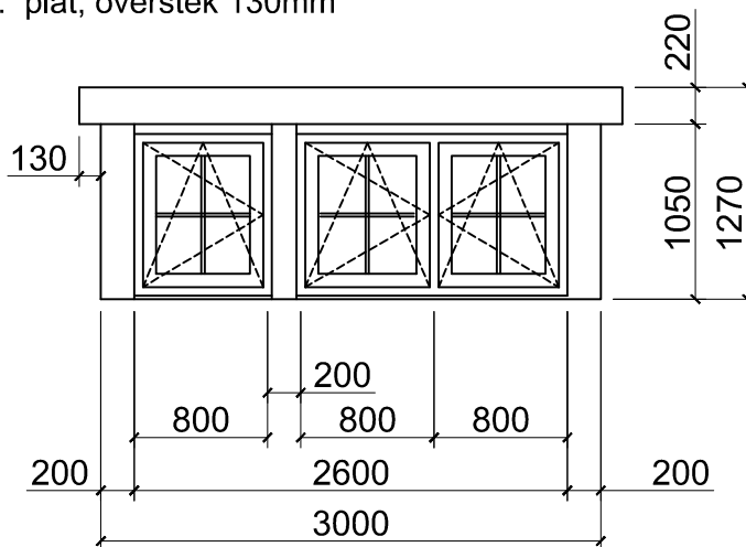
AANZICHT DAKKAPEL VOORGEVEL (schaal 1:50)
