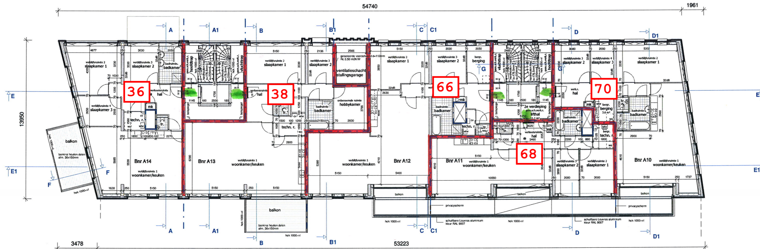
2e verdieping
