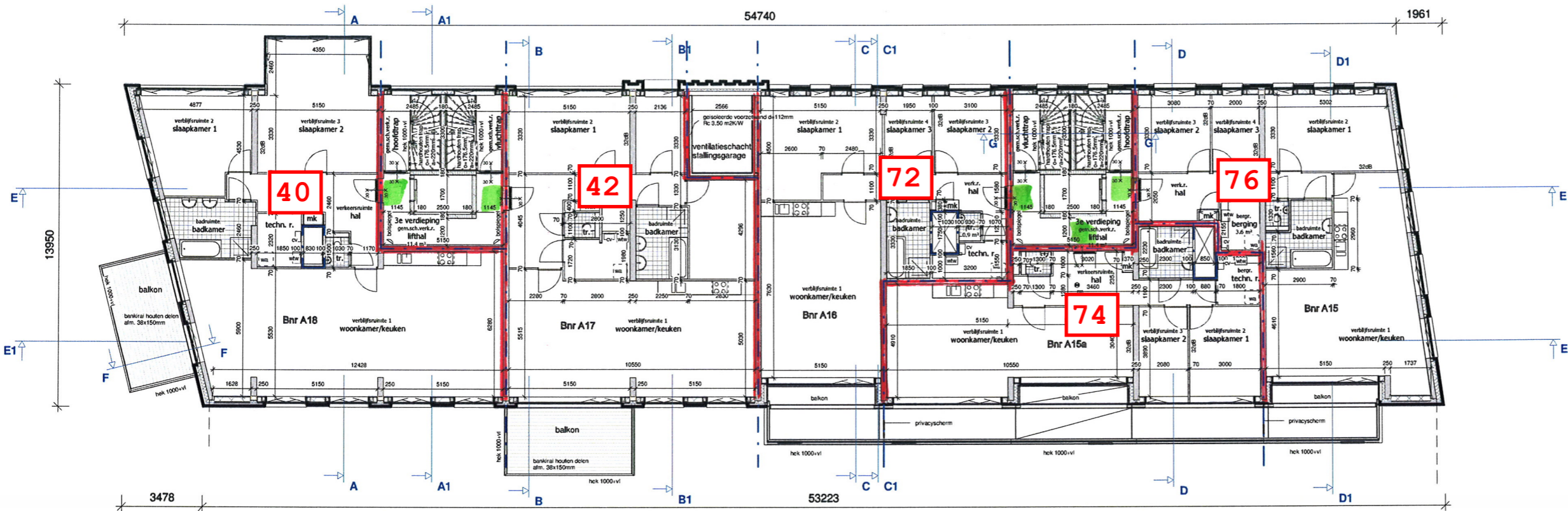
3e verdieping
