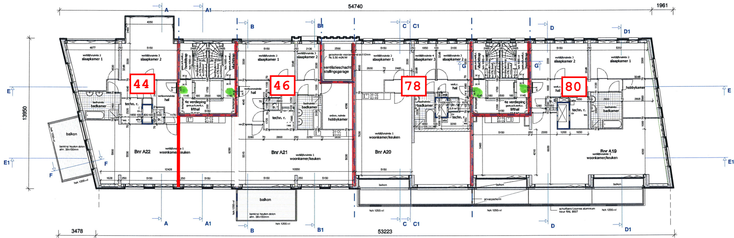
4e verdieping
