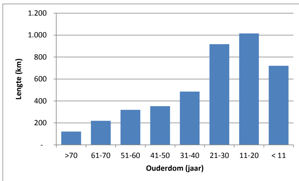
Figuur 4: Leeftijdsopbouw van de Amsterdamse riolering
