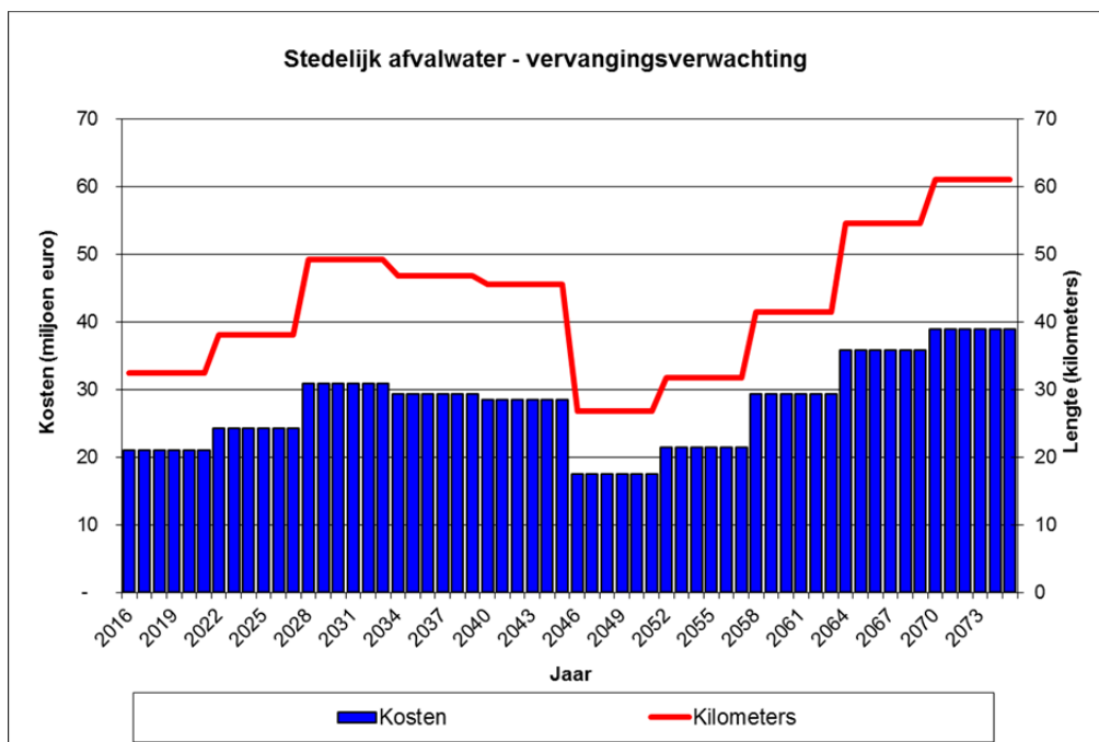
Figuur 6: Vervangingsverwachting vuilwaterriolering
