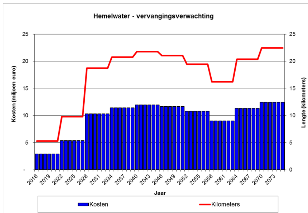
Figuur 8: Vervangingsverwachting hemelwaterriolering
