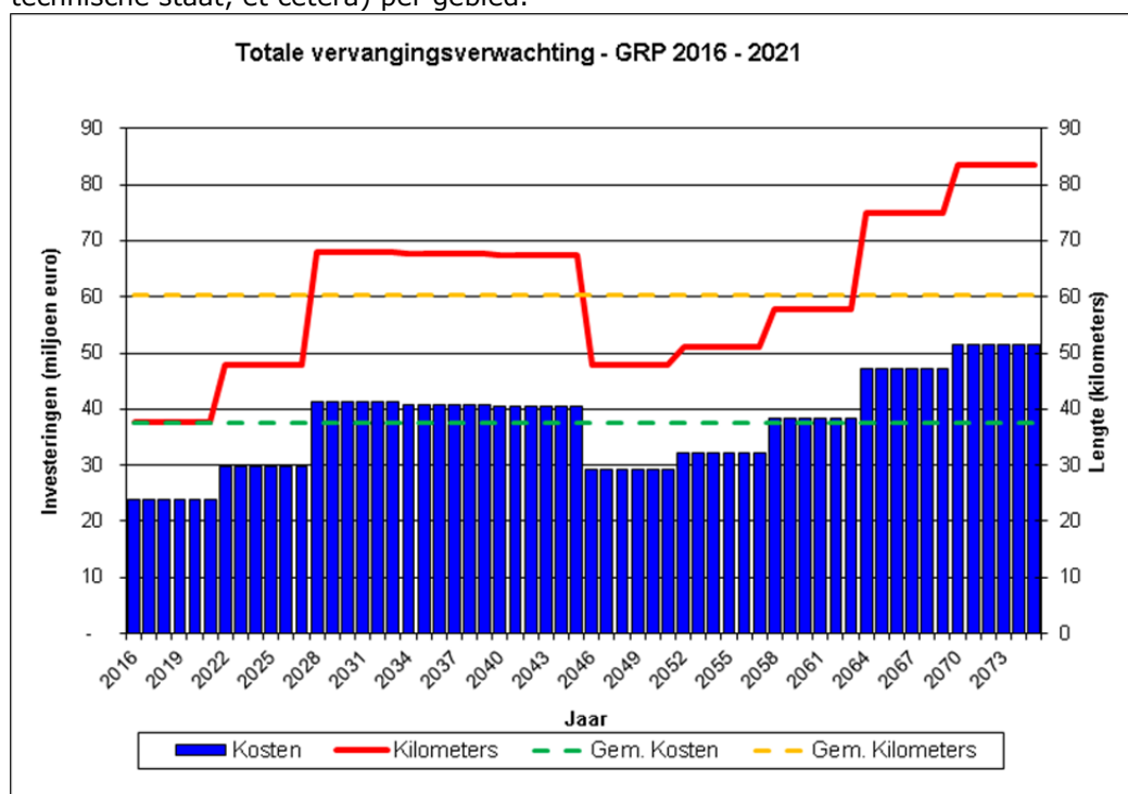
Figuur 9: Totale vervangingsverwachting (stedelijk afval- en hemelwater)
