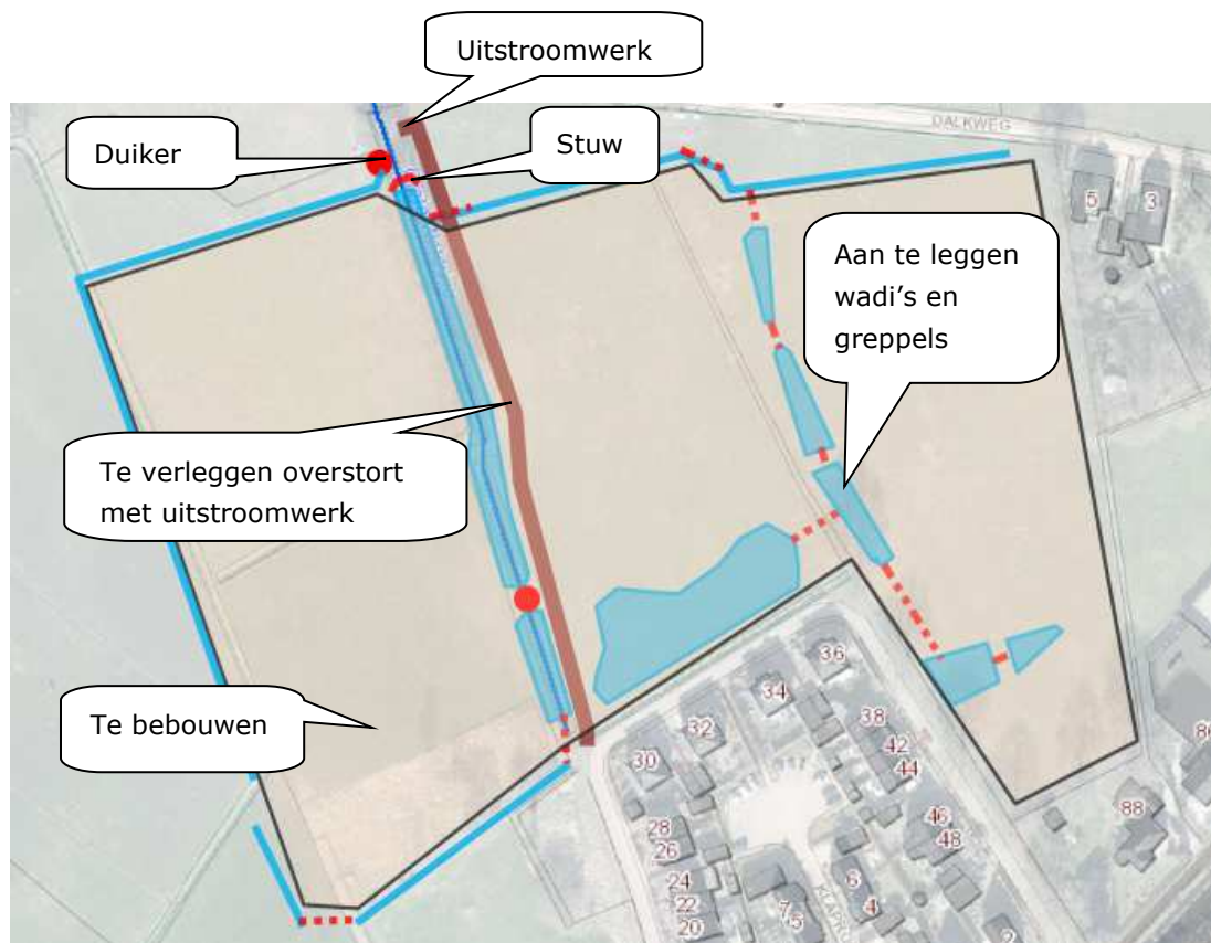
Aan te leggen oppervlaktewaterlichamen C (wadi's/greppels), duikers, stuw en te verleggen overstort.
