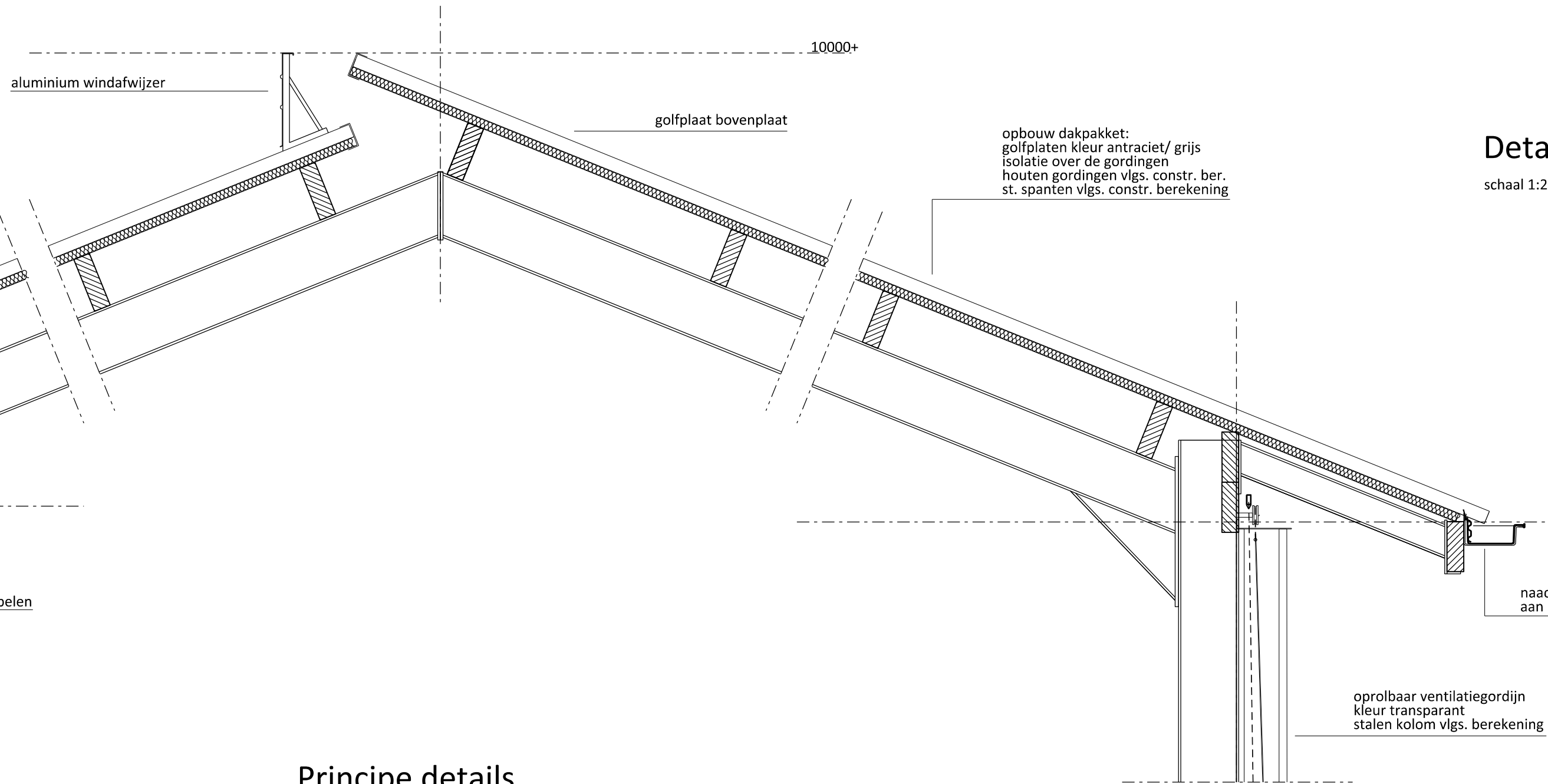
Detail 3 schaal 1:20
