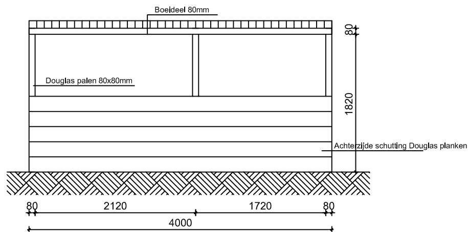
Nieuw achteraanzicht
