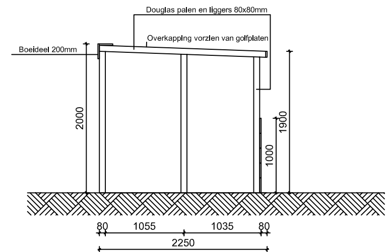
Nieuwe doorsnede A-A
