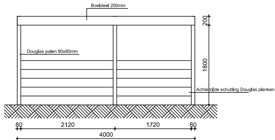
Nieuw vooraanzicht
