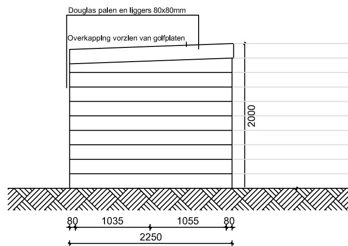
Linker zijgevel
