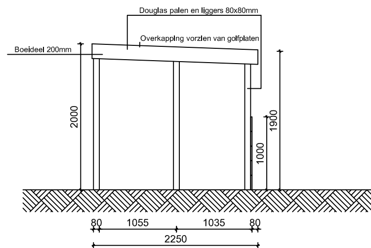
Rechter zijgevel
