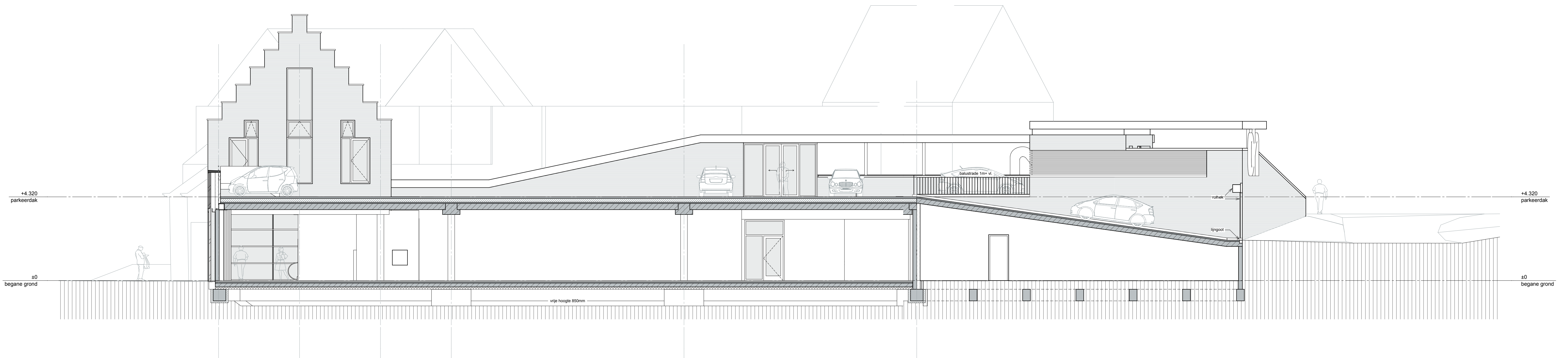
doorsnede J-J
