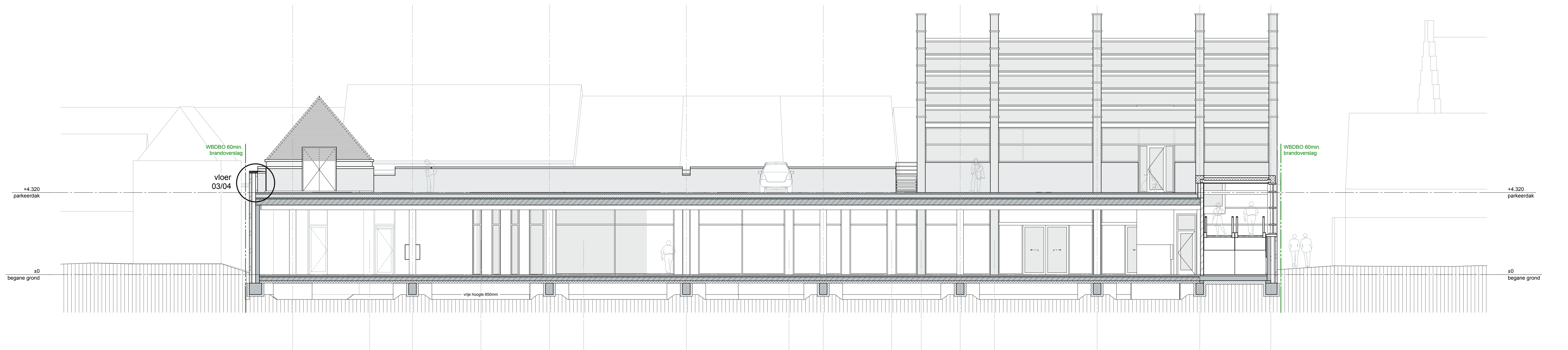
doorsnede C-C
