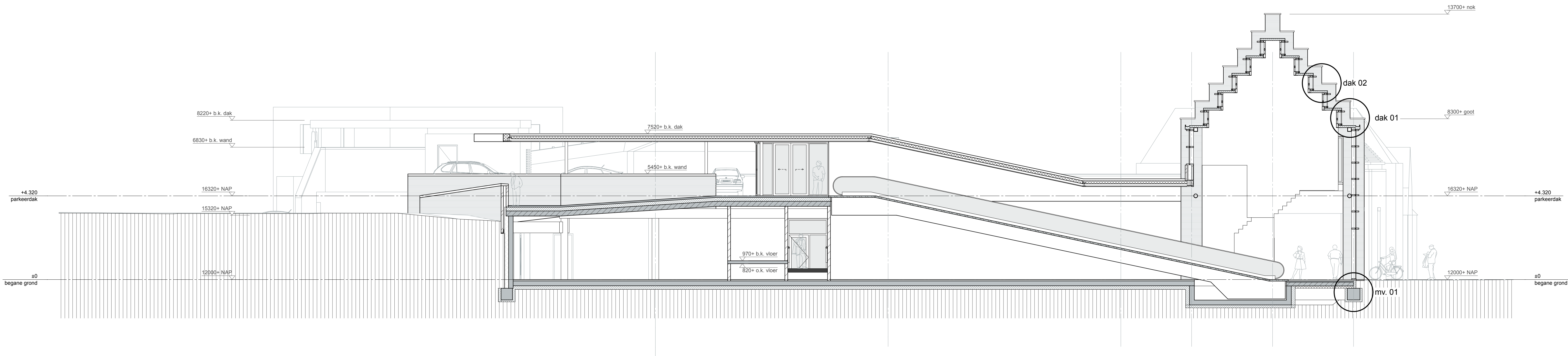
doorsnede B-B
