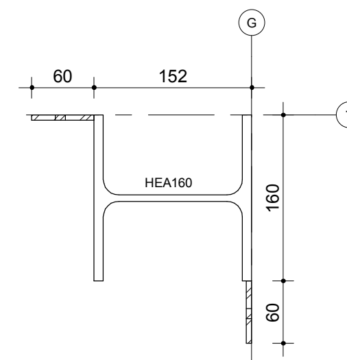
Detail t.b.v. bevestiging prefab paneel 1:5
