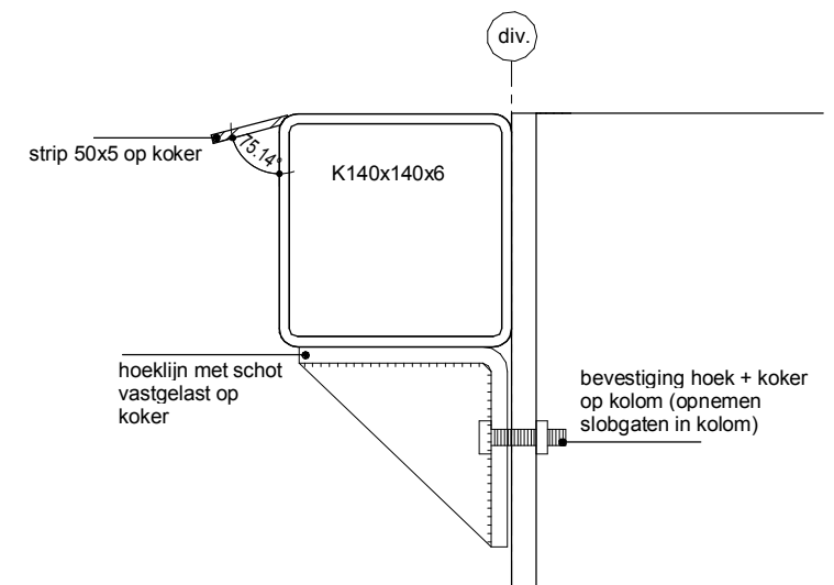
Detail t.p.v. alle liggers L3 - 1:5
