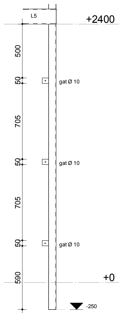
vooraanzicht t.b.v. bevestiging prefab paneel 1:20
