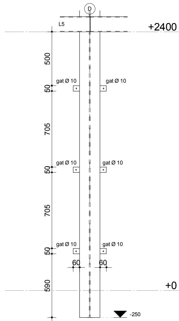
vooraanzicht t.b.v. bevestiging prefab paneel 1:20
