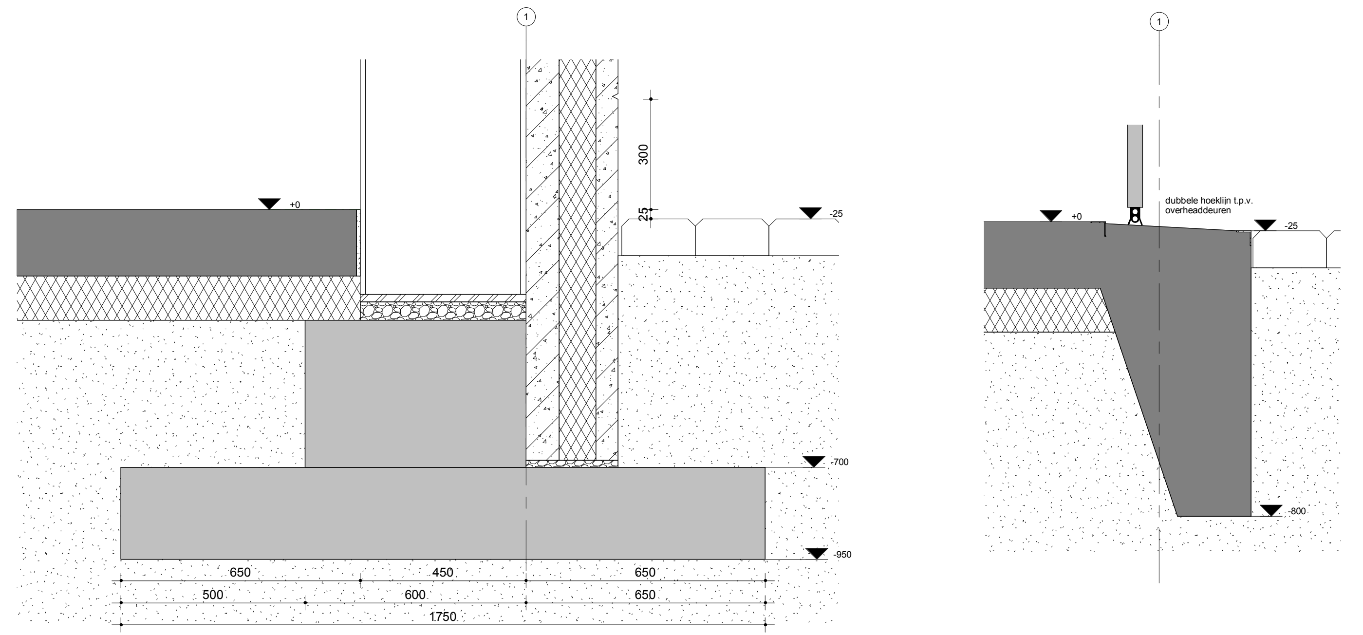
Detail F1A
