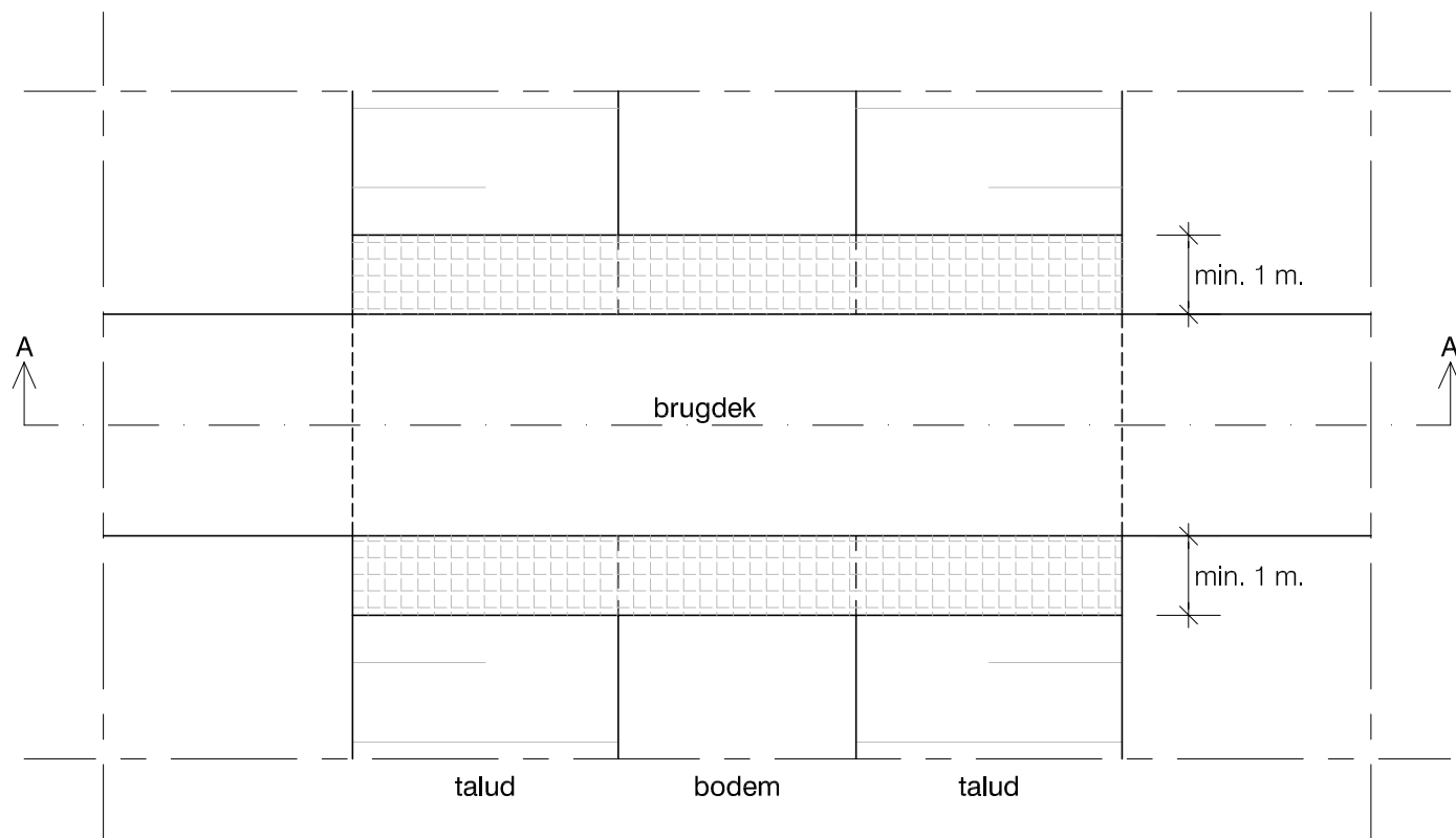
Bovenaanzicht
